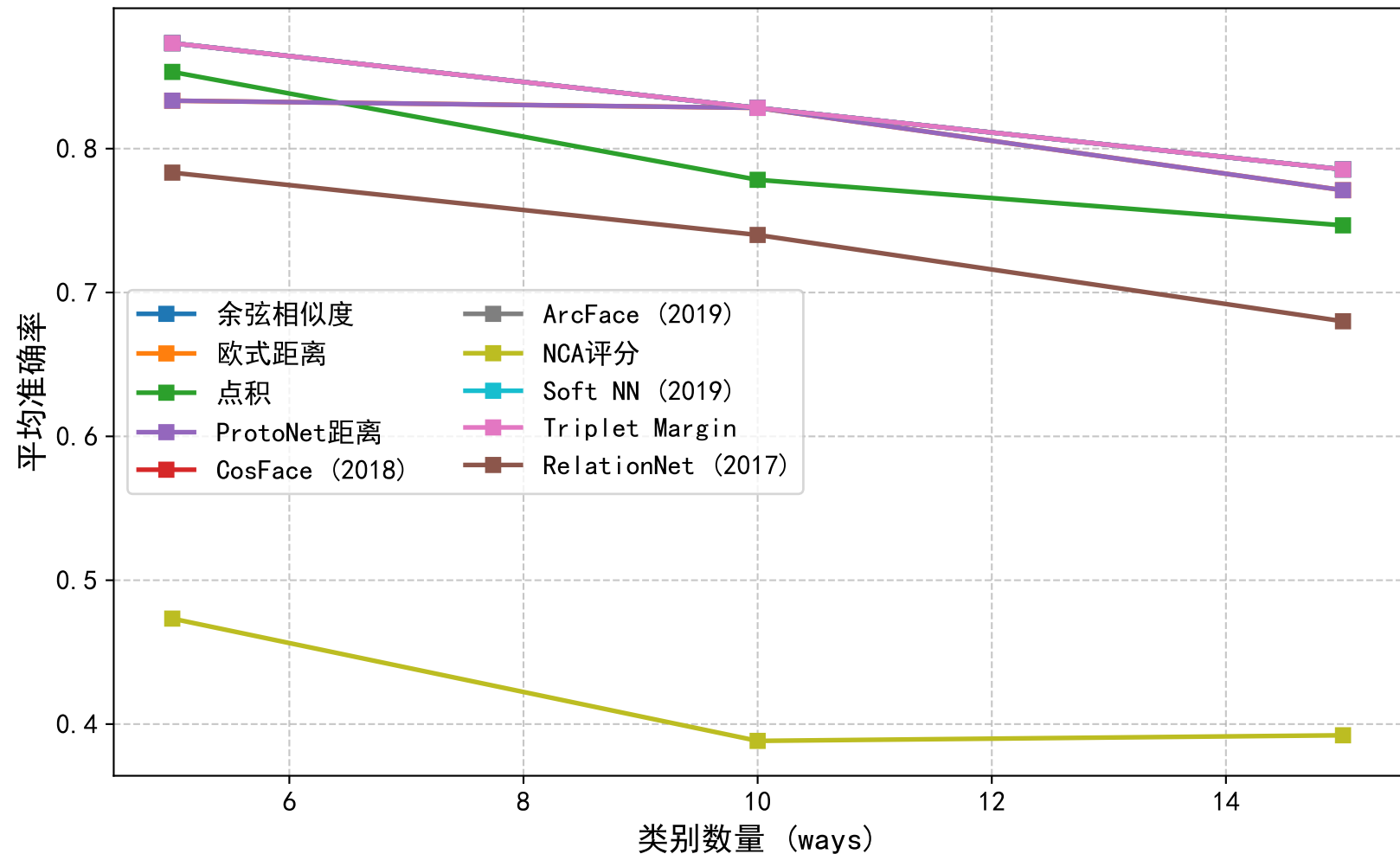
类别数量对不同评分函数的影响
