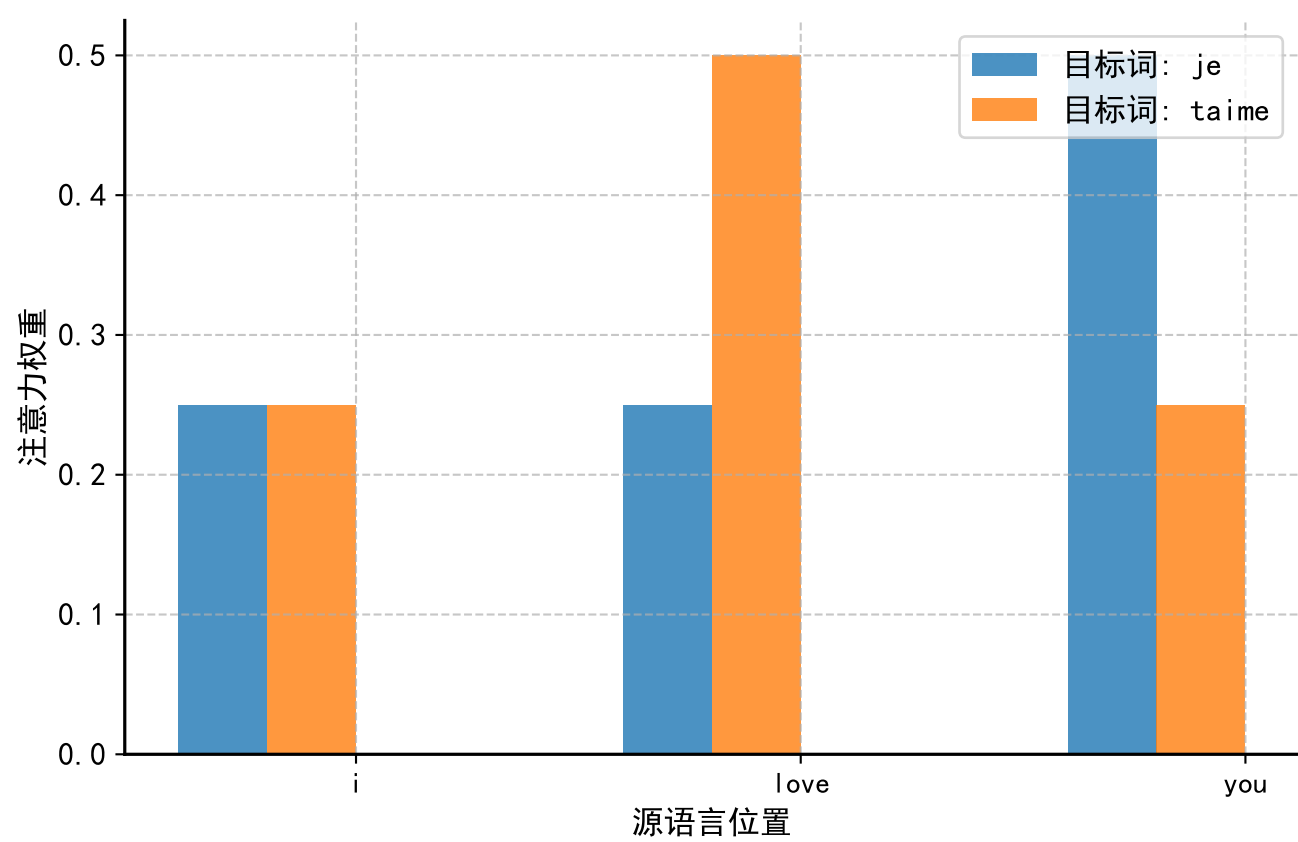
各目标词的注意力分布
