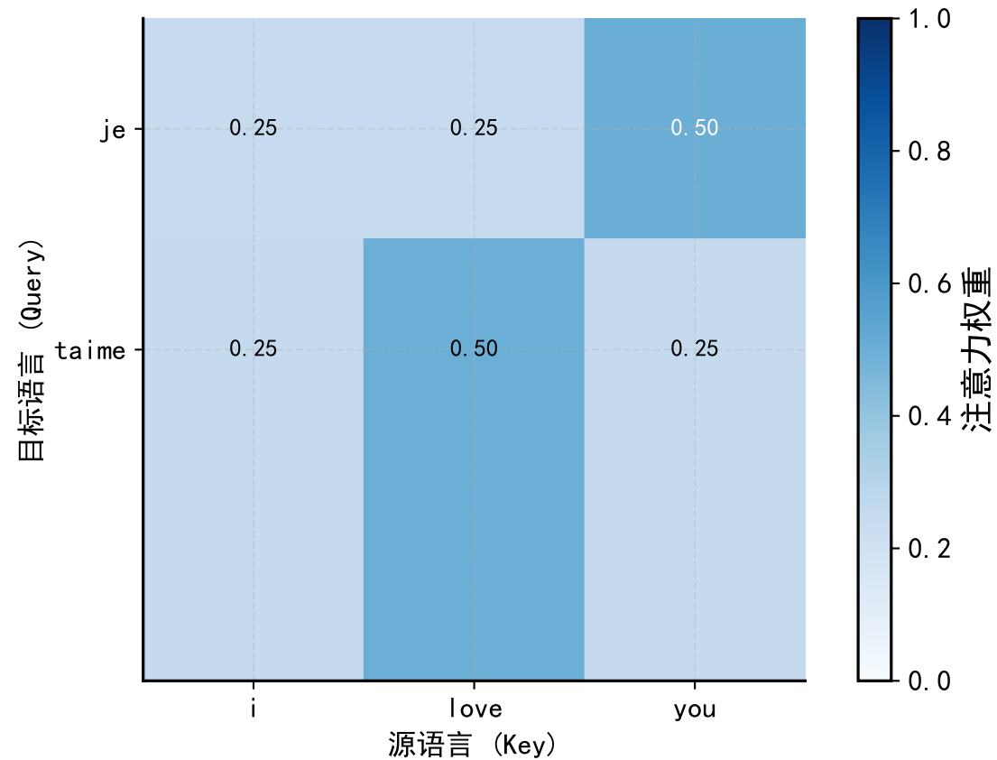
真实注意力权重（平均所有头）
