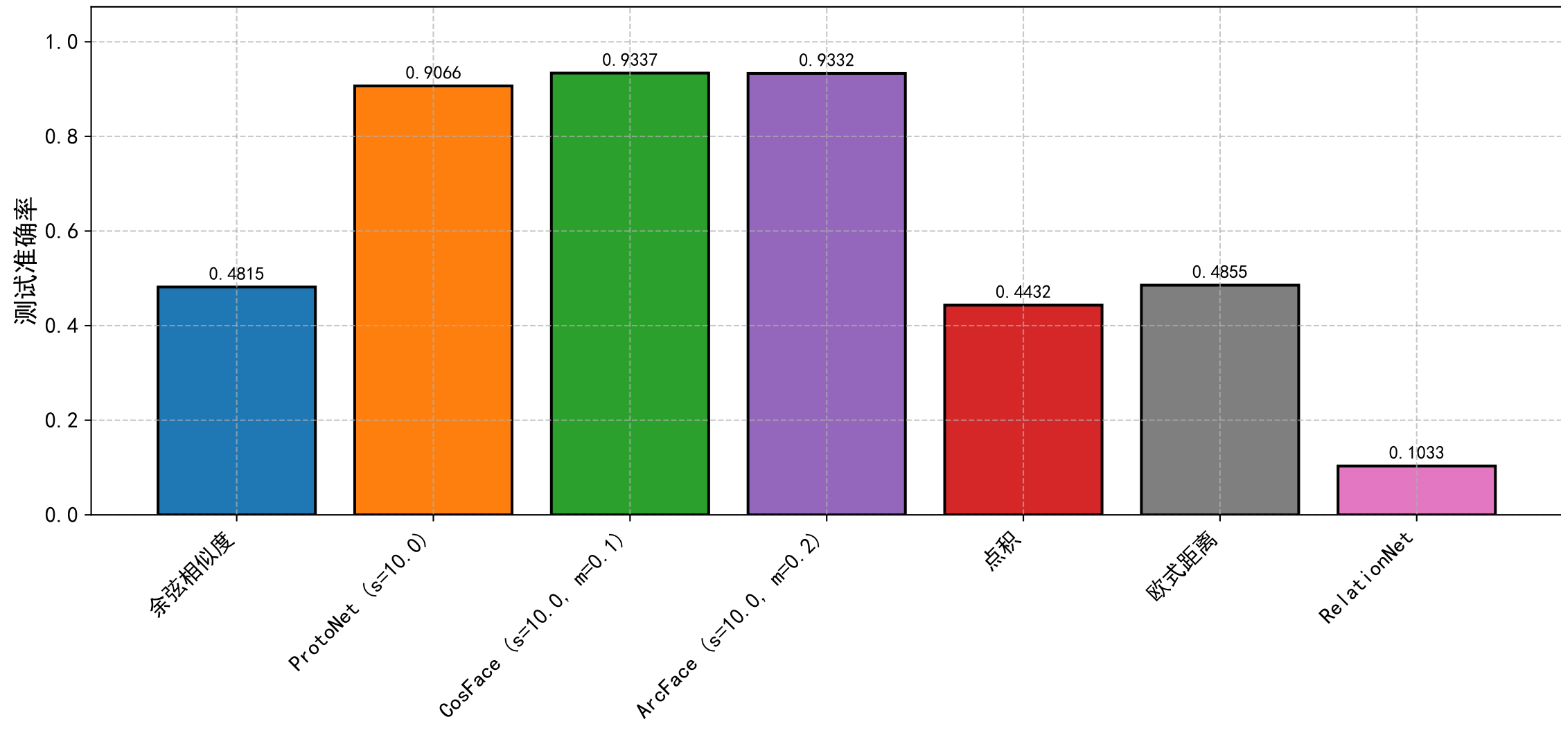
各评分函数最终测试准确率对比
