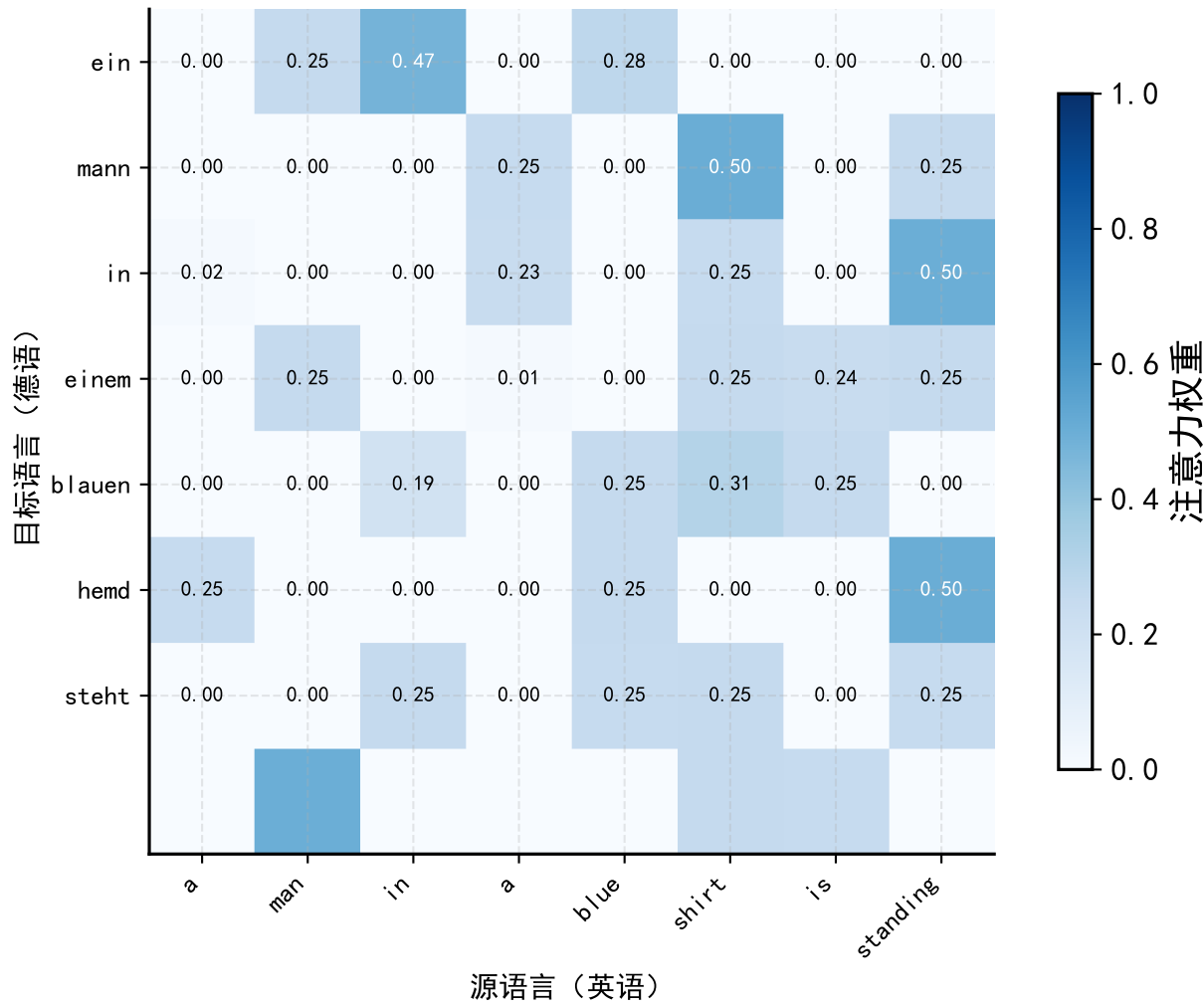
翻译注意力权重热力图 (英→德)
