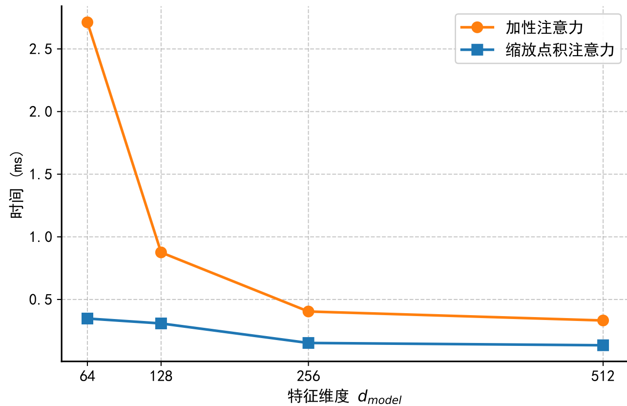
计算时间 vs 特征维度
