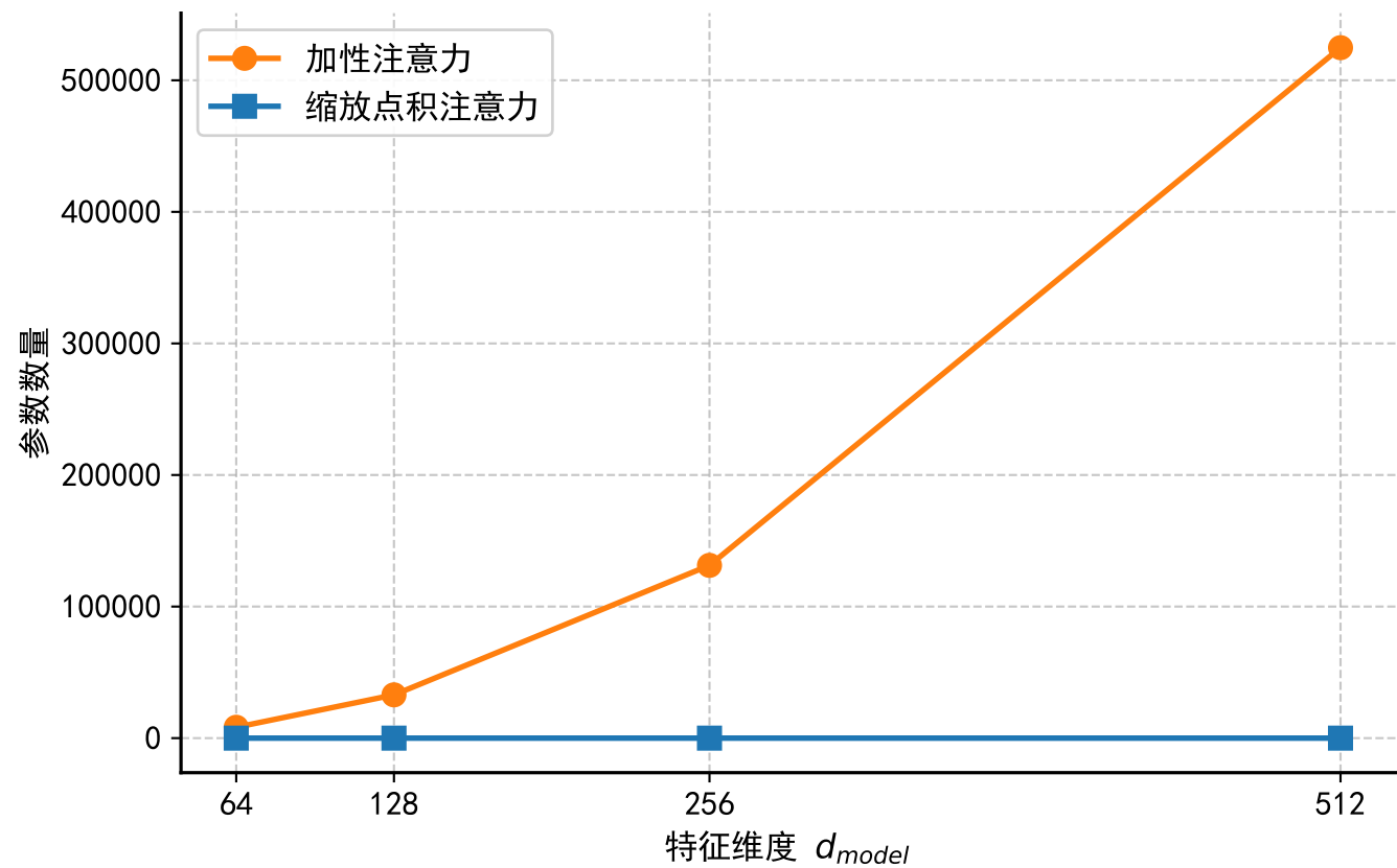
参数数量 vs 特征维度
