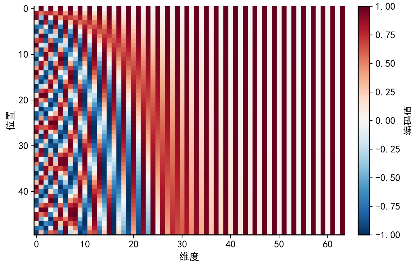
正弦余弦位置编码
