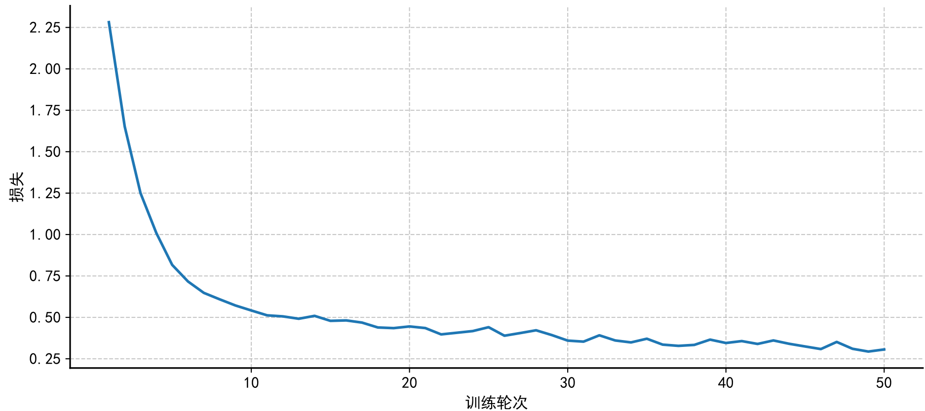
字符级语言模型训练损失
