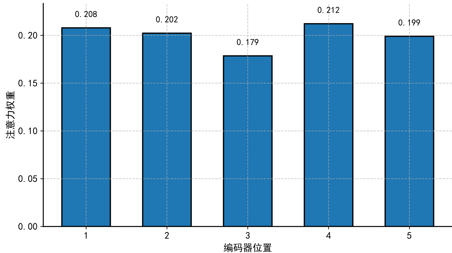
Bahdanau注意力权重分布
