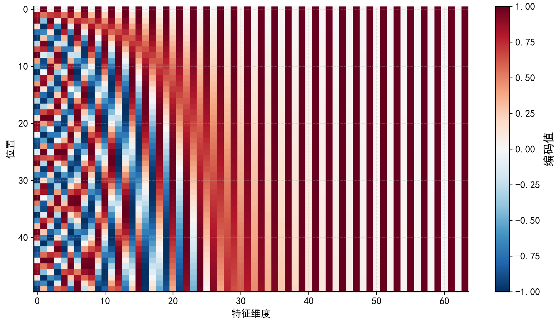
Transformer位置编码
