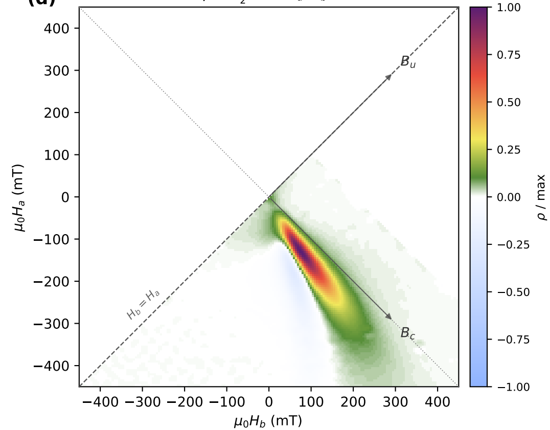
(d) FORC distribution \rho = -\frac{1}{2} \partial^2 M / \partial H_a \partial H_b
