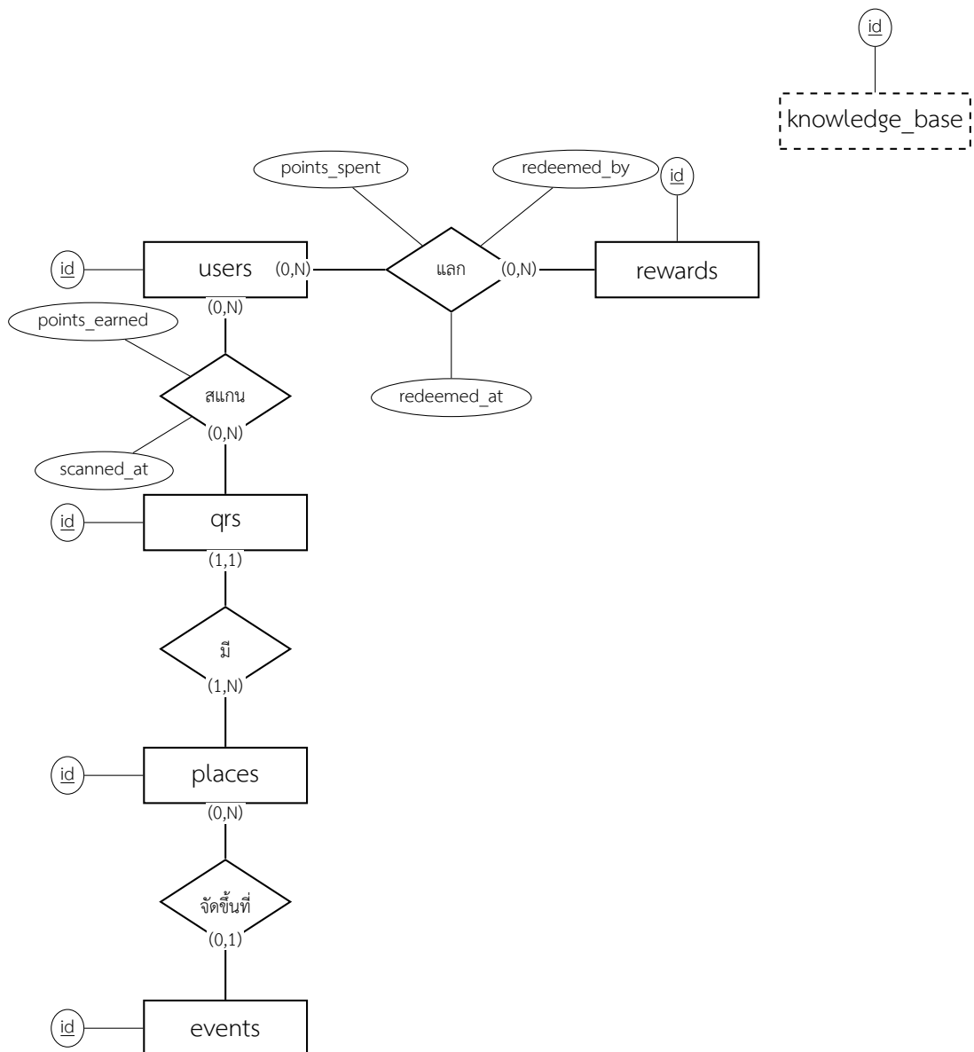
ภาพที่ 30 E-R Diagram (Chen Notation) แสดงความสัมพันธ์ระหว่าง Entity ในฐานข้อมูล
