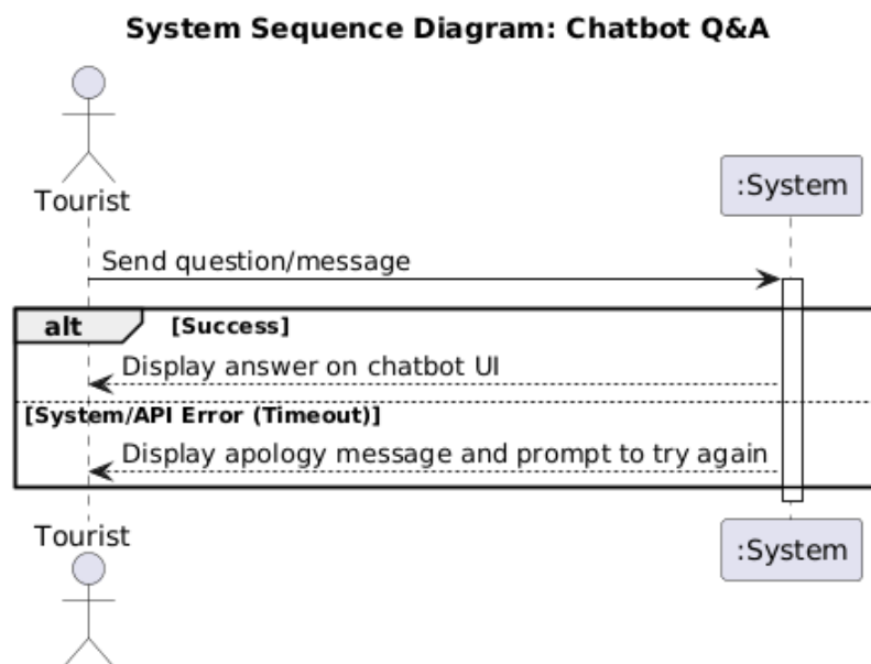
ภาพที่ 16 System Sequence Diagram: ฟังก์ชันถามตอบข้อมูลโดยใช้แชตบอต
