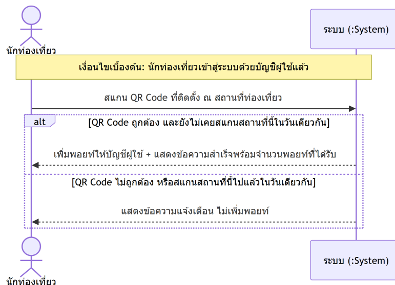
ภาพที่ 19 System Sequence Diagram: สแกน QR สะสมพอยท์
