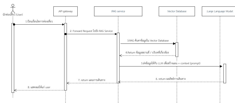
ภาพที่ 23 Detailed Sequence Diagram: การสร้างแผนการเดินทางด้วย RAG และ LLM
