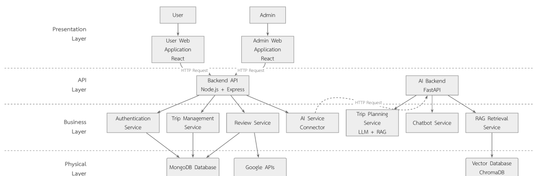
ภาพที่ 24 สถาปัตยกรรมของระบบ
