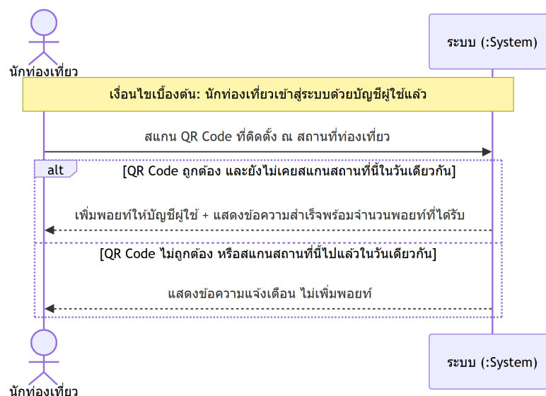
ภาพที่ 21 System Sequence Diagram: สแกน QR สะสมพอยท์
