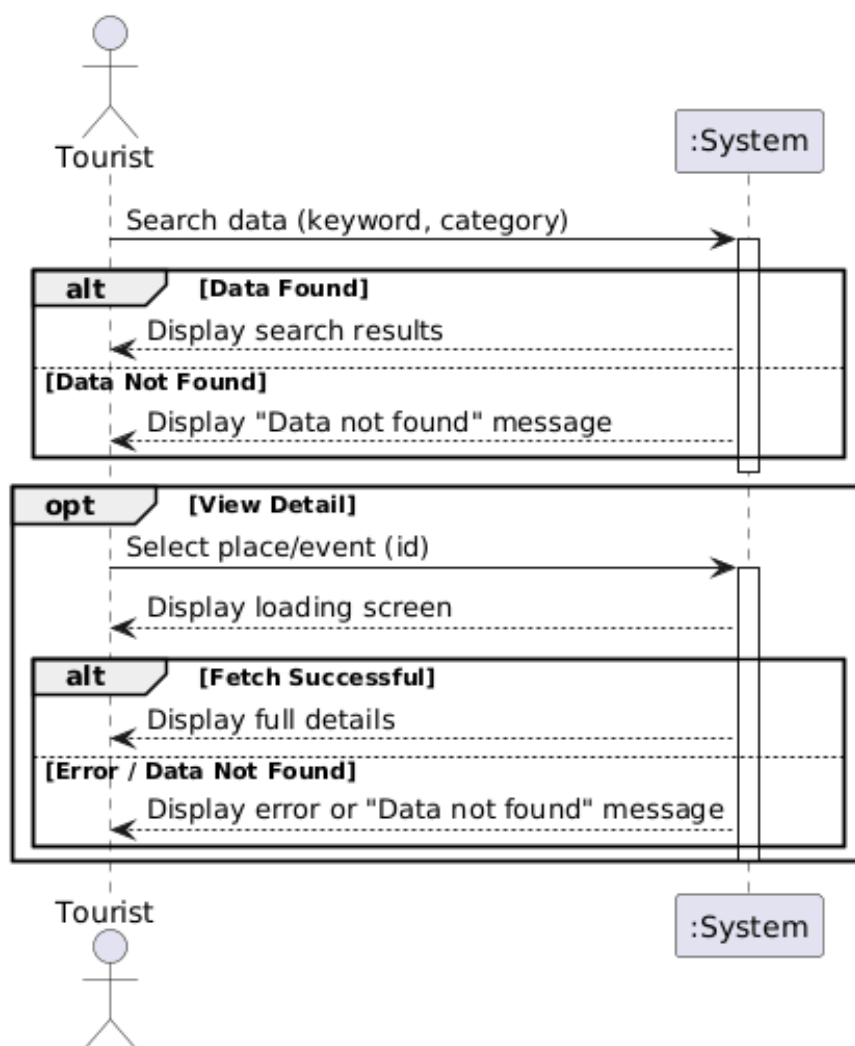
ภาพที่ 17 System Sequence Diagram: ฟังก์ชันค้นหาข้อมูลสถานที่และกิจกรรม
