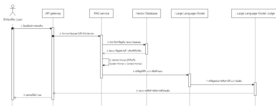
ภาพที่ 25 Detailed Sequence Diagram: การสร้างแผนการเดินทางด้วย RAG และ LLM
