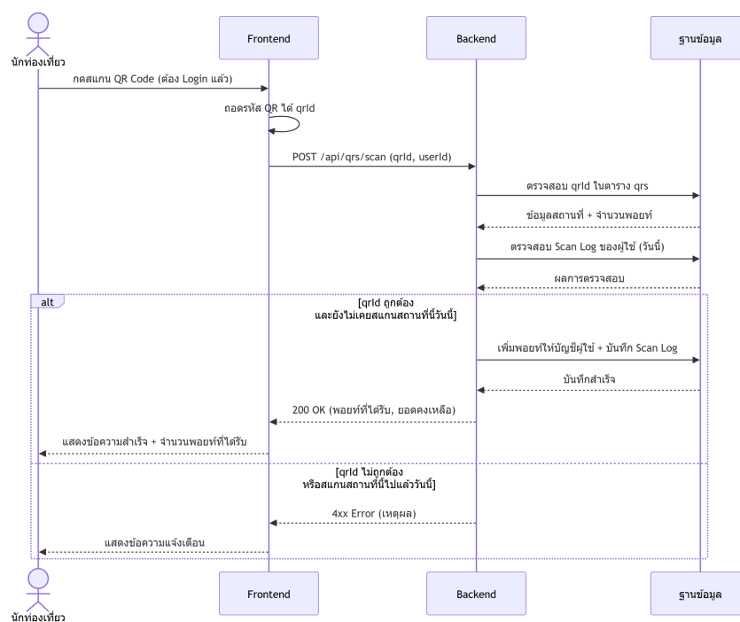
ภาพที่ 28 Detailed Sequence Diagram: สแกน QR สะสมพอยท์
