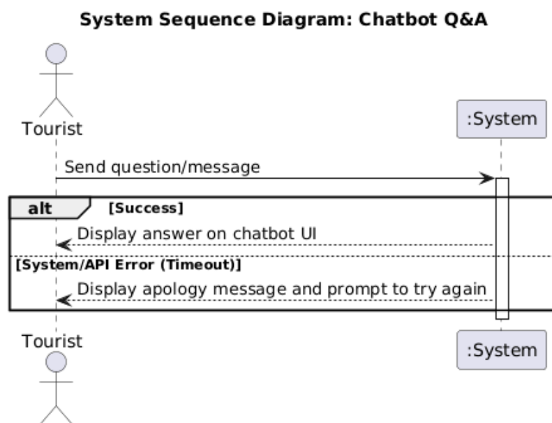
ภาพที่ 16 System Sequence Diagram: ฟังก์ชันถามตอบข้อมูลโดยใช้แชทบอต
