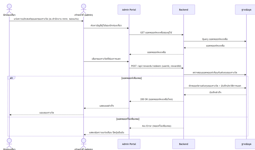
ภาพที่ 29 Detailed Sequence Diagram: แลกของรางวัล ณ สำนักงาน ททท. ขอนแก่น
