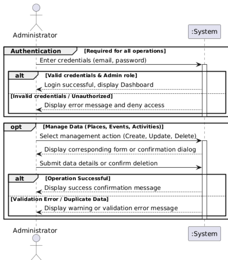
ภาพที่ 19 System Sequence Diagram: การเข้าสู่ระบบและจัดการข้อมูลมาตรฐาน
