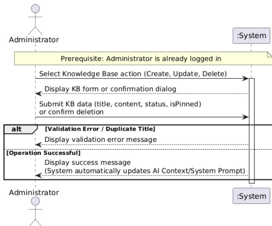
ภาพที่ 20 System Sequence Diagram: การจัดการฐานความรู้ (Knowledge Base)
