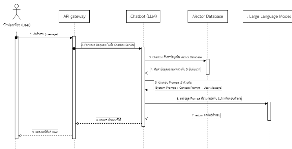
ภาพที่ 26 Detailed Sequence Diagram: การทำงานของระบบผู้ช่วยเสมือน (แชทบอต)
