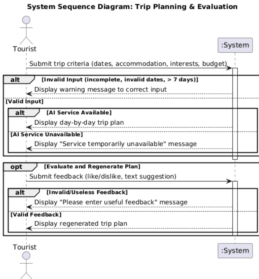
ภาพที่ 18 System Sequence Diagram: ฟังก์ชันสร้างแผนการเดินทาง
