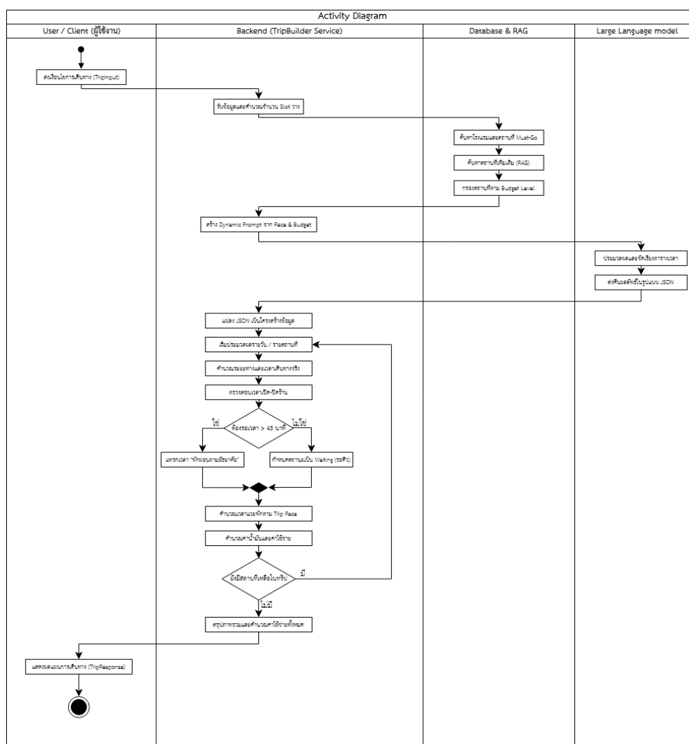
ภาพที่ 23 Activity Diagram ตรรกะการประมวลผลเพื่อสร้างแผนการเดินทาง
