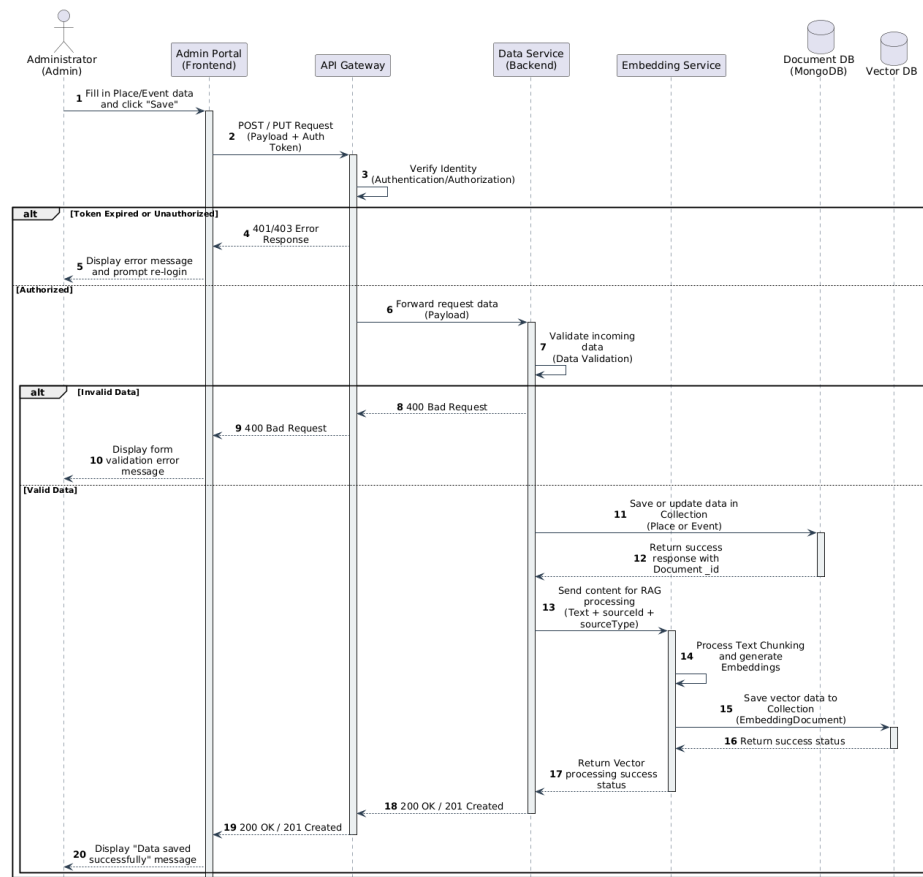
ภาพที่ 27 Detailed Sequence Diagram สำหรับผู้ดูแลระบบ
