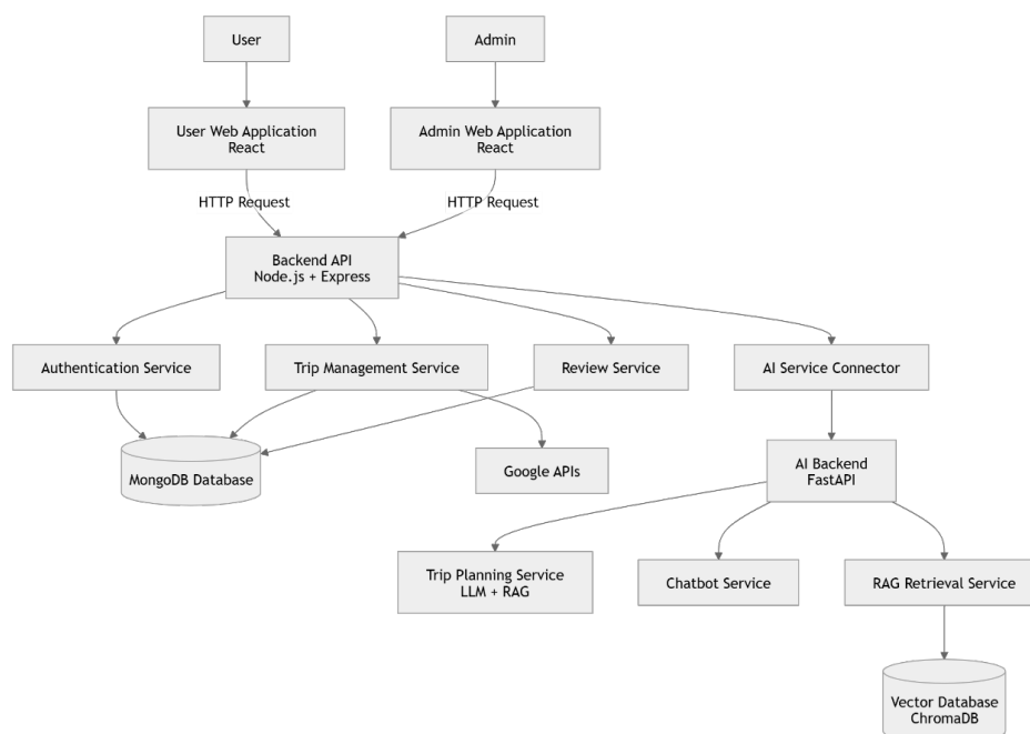
ภาพที่ 24 สถาปัตยกรรมของระบบ
