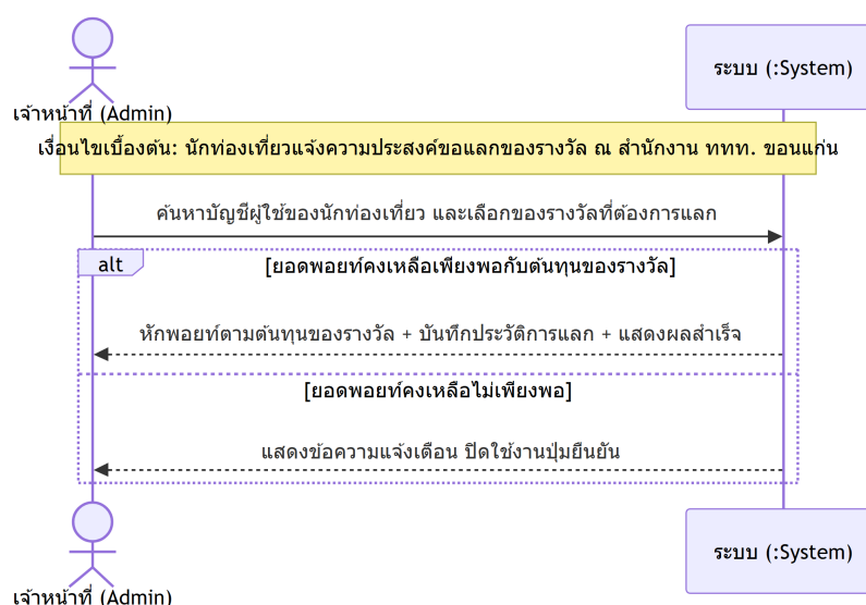
ภาพที่ 22 System Sequence Diagram: แลกของรางวัล ณ สำนักงาน ททท. ขอนแก่น
