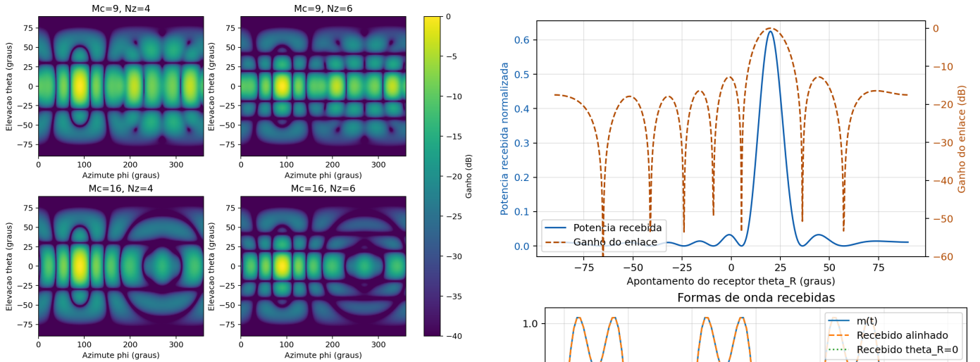
Figura 5. Mapas bidimensionais do arranjo cilíndrico para todas as combinações de M_c e N_z .
