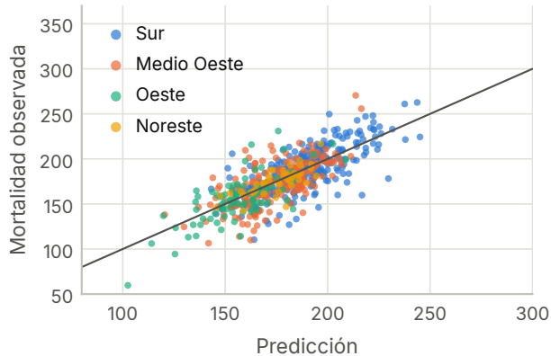
Prueba: Ridge
