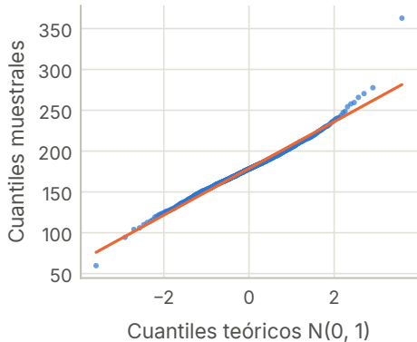
Gráfico Q-Q normal
