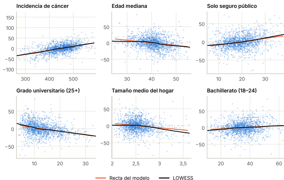
Figura 7.2: Residuos parciales de las seis explicativas con mayor efecto: la recta es la contribución estimada por el modelo y la curva, un suavizado LOWESS de los puntos.
