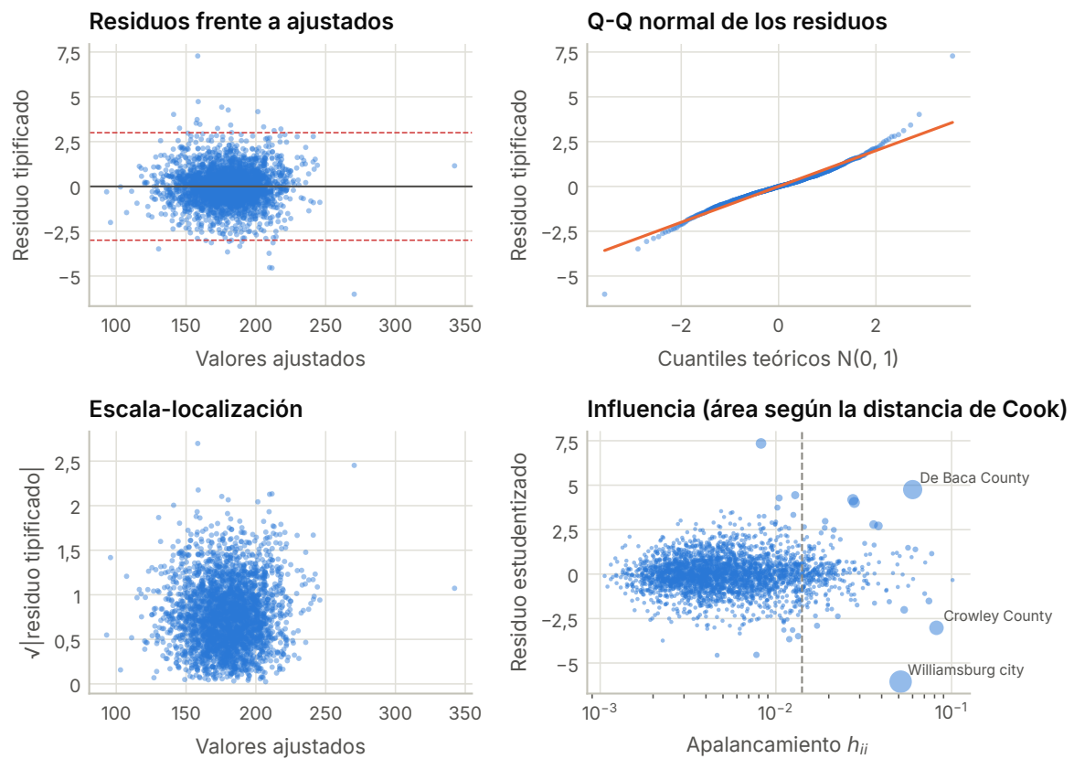
Figura 7.1: Gráficos de diagnóstico del modelo final: residuos tipificados frente a valores ajustados, gráfico cuantil-cuantil normal, escala-localización y residuos estudentizados frente al apalancamiento (el área de cada punto es proporcional a la distancia de Cook).
