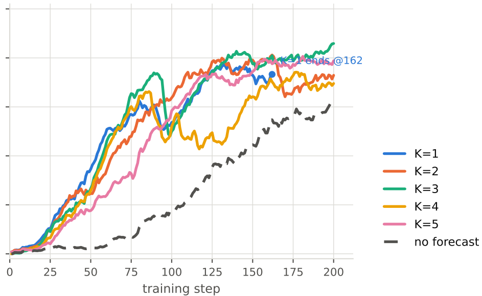
EMA span 20
