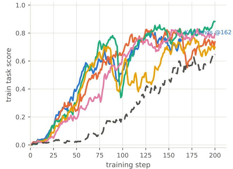
EMA span 10
