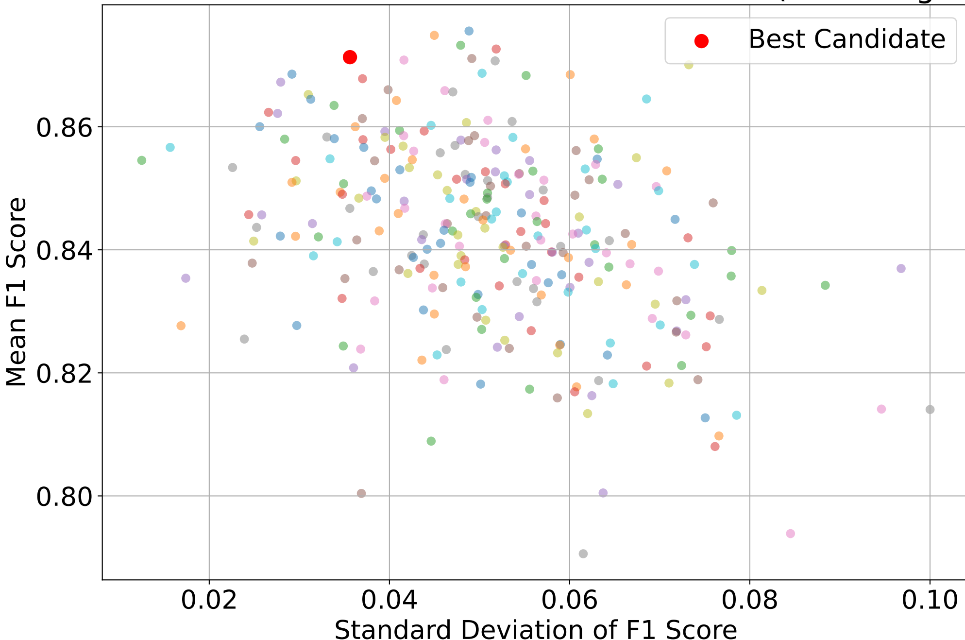
Mean F1 Score vs Standard Deviation of F1 Score (All Configurations)
