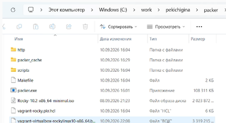
Рис. 4: Рабочий каталог
