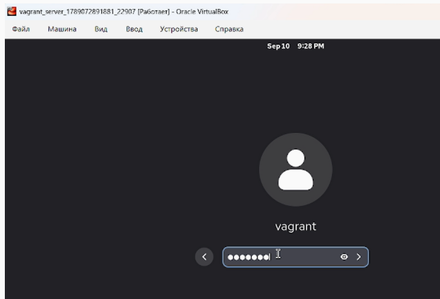
Рис. 6: Вводим пароль
