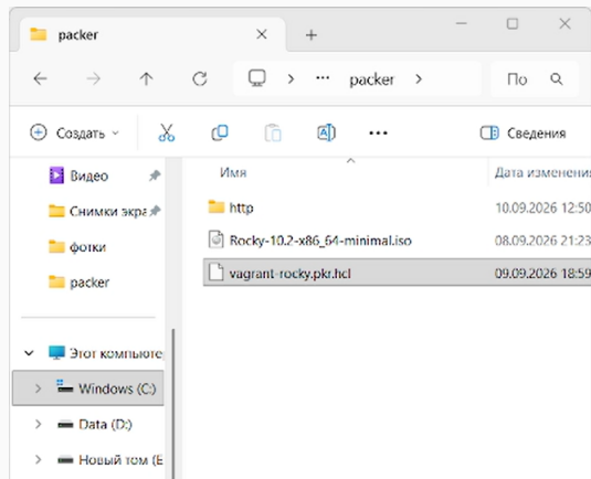
Рис. 1: Подкаталог packer
