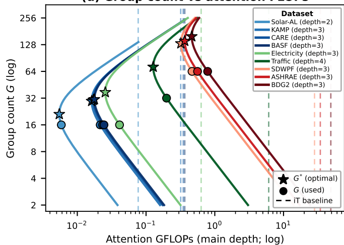
(d) Group count vs attention FLOPs
