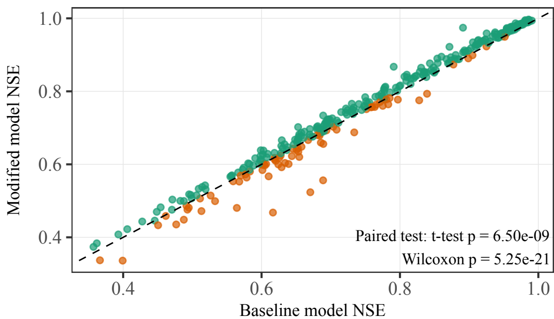
(d) Station-wise NSE comparison
