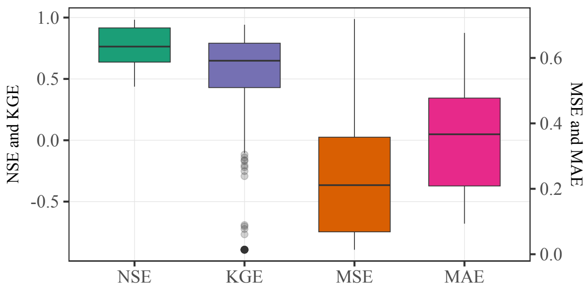
(d) Station-wise NSE comparison
