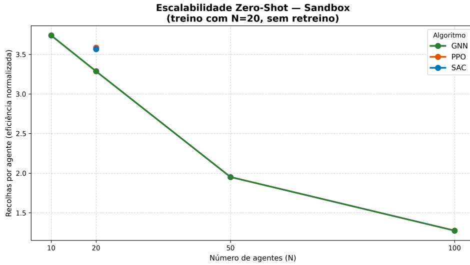
FIGURA 6.22. Degradação (ou instabilidade) do desempenho com o aumento do número de agentes, sem retreino.
