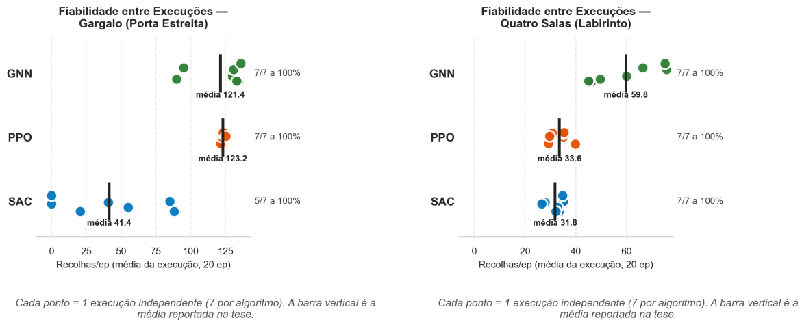
FIGURA 6.13. Recolhas/ep por execução: Gargalo (esq.) e Quatro Salas (dir.).
