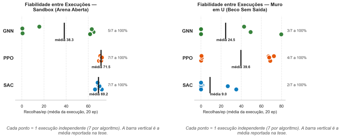
FIGURA 6.12. Recolhas/ep por execução (7 execuções, 20 ep cada): Sandbox (esq.) e Muro em U (dir.). Cada ponto é uma execução independente e a barra vertical é a média reportada na tese; note-se que os dois painéis têm escalas horizontais diferentes.
