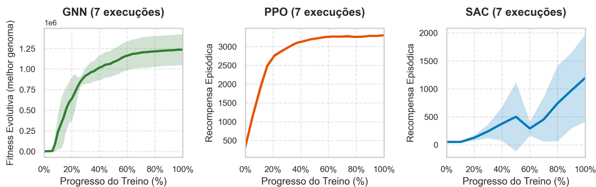
Curvas de Aprendizagem — Gargalo (Porta Estreita)
