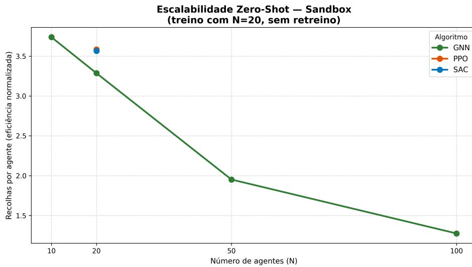
FIGURA 6.22. Degradação (ou estabilidade) do desempenho com o aumento do número de agentes, sem retreino.
