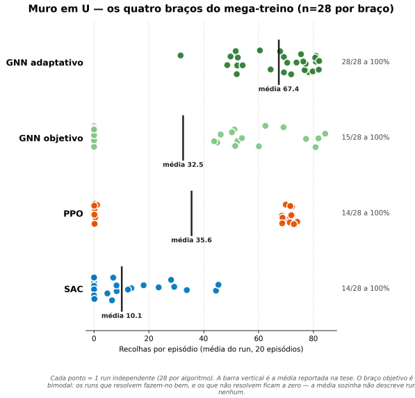
Figura 3: As 28 execuções independentes de cada braço no Muro em U. Cada ponto é uma execução (média de 20 episódios determinísticos); a barra vertical é a média. A leitura decisiva não é a diferença de médias, mas a forma das distribuições: os três braços sem anilamento da novidade repartem-se entre execuções que resolvem o cenário e execuções que ficam a zero, praticamente sem nada pelo meio, enquanto a dosagem adaptativa não deixa uma única execução por resolver.
