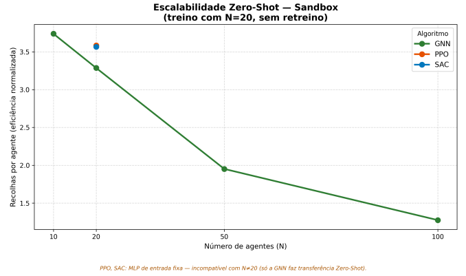
Figura 4: Transferência zero-shot no cenário Sandbox para tamanhos de enxame nunca vistos ( N \in \{10, 20, 50, 100\} ), sem retreino. O eixo vertical é a recolha per capita : a sua descida ( 3,74 \rightarrow 1,27 ) reflete a partilha de um recurso finito por mais agentes — as recolhas totais crescem ( 37,4 \rightarrow 127,3 ) e a taxa de sucesso mantém-se em 100%. Nos sete cenários da bateria o sucesso é 100% em todas as 28 combinações, com retenção per capita de 58–90% nos cenários com paredes. O PPO/SAC, com entrada de dimensão fixa, são incompatíveis com N \neq 20 e surgem como pontos isolados.
