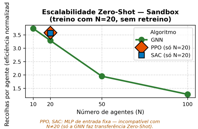
Figura 4: Transferência zero-shot no cenário Sandbox para tamanhos de enxame nunca vistos ( N \in \{10, 20, 50, 100\} ), sem treino. O eixo vertical é a recolha per capita : a sua descida ( 3,74 \rightarrow 1,27 ) reflete a partilha de um recurso finito por mais agentes — as recolhas totais crescem ( 37,4 \rightarrow 127,3 ) e a taxa de sucesso mantém-se em 100%. Nos sete cenários da bateria o sucesso é 100% em todas as 28 combinações, com retenção per capita de 58–90% nos cenários com paredes. O PPO/SAC, com entrada de dimensão fixa, são incompatíveis com N \neq 20 e surgem como pontos isolados.
