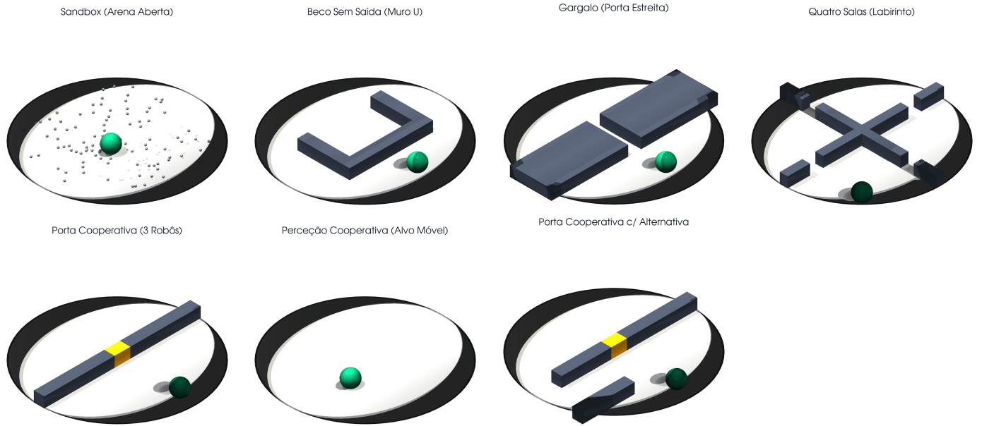
Figura 1: Os sete cenários de avaliação, renderizados a partir da geometria real do simulador. Em cima: Sandbox (aberto, com obstáculos esféricos), Beco Sem Saída (Muro em U), Gargalo e Quatro Salas. Em baixo: Porta Cooperativa (passagem a âmbar, abre com \geq 3 agentes), Percepção Cooperativa (alvo móvel) e Porta Cooperativa com Alternativa (cenário deceptive : a porta atrai, o corredor lateral resolve). O ninho é a esfera verde.
