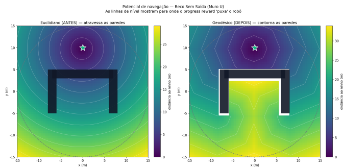
Figura 2: Potencial de recompensa no Muro em U: a distância euclidiana (esquerda) atravessa a parede e induz um mínimo local; o campo geodésico (direita), calculado por Dijkstra sobre a grelha com obstáculos dilatados, premeia o contorno e elimina a armadilha. É um sinal de treino, não uma observação.
