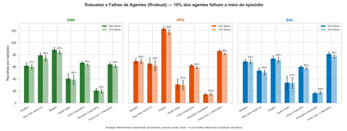
Figura 7: Retenção de desempenho sob falha de 10% dos agentes a meio do episódio, relativa à execução nominal (mesmas seeds). Os três painéis partilham a escala vertical, pelo que as alturas são comparáveis entre paradigmas. Nenhum paradigma colapsa; a redundância emerge da partilha de parâmetros e da observação puramente local.
