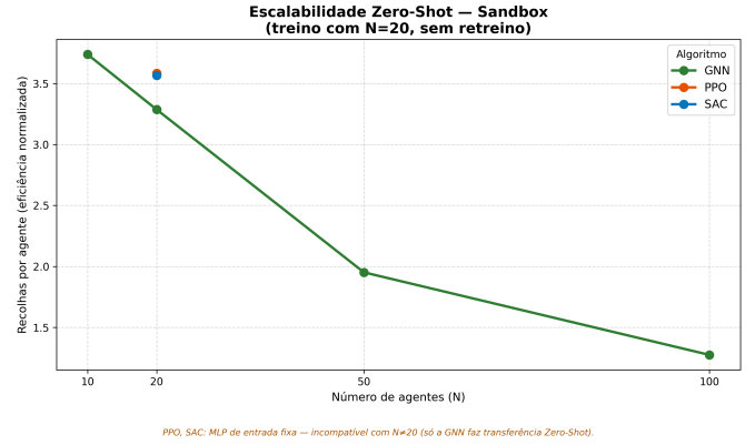
Figura 6: Transferência zero-shot no cenário Sandbox para tamanhos de enxame nunca vistos ( N \in \{10, 20, 50, 100\} ), sem retreino. O eixo vertical é a recolha per capita : a sua descida (3,74 \rightarrow 1,27) reflete a partilha de um recurso finito por mais agentes — as recolhas totais crescem (37,4 \rightarrow 127,3) e a taxa de sucesso mantém-se em 100%. Nos sete cenários da bateria o sucesso é 100% em todas as 28 combinações, com retenção per capita de 58–90% nos cenários com paredes. O PPO/SAC, com entrada de dimensão fixa, são incompatíveis com N \neq 20 e surgem como pontos isolados.
