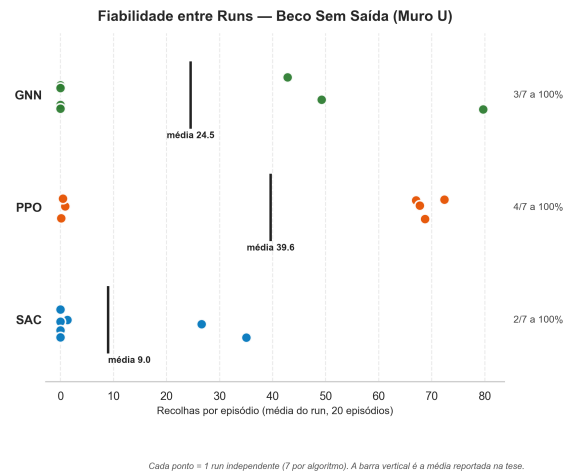
Figura 4: Recolhas por episódio no Muro em U: um ponto por execução de treino (média dos 20 episódios determinísticos dessa execução) e a barra vertical na média do braço. A dispersão não é ruído de avaliação — reflete execuções que resolvem integralmente o cenário e execuções que falham por completo. Com n = 7 mostram-se as execuções uma a uma: um diagrama de caixa a cobrir todo o intervalo sugeriria densidade onde não existe uma única execução.
