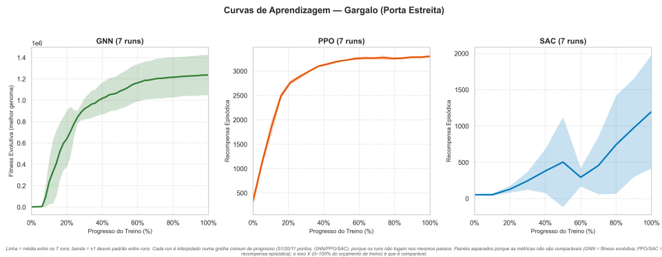
FIGURA 6.7. Curvas de aprendizagem no cenário Gargalo.
