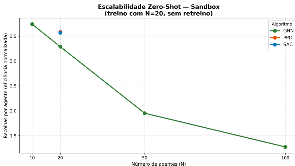
FIGURA 6.22. Eficiência por agente (recolhas por episódio a dividir pelo número de agentes) com o aumento do enxame, sem retreino, no cenário Sandbox. Só a linha do controlador de grafo atravessa toda a gama: o PPO e o SAC têm um único ponto, em N = 20 , porque a política MLP de entrada fixa não admite outras dimensões de enxame.
