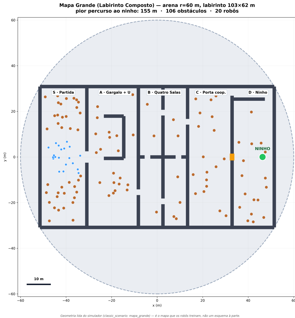
FIGURA 7.1. Planta do mapa grande, lida da geometria do próprio simulador: cinco zonas de oeste para este, 106 obstáculos, ninho na câmara a este e caixa de spawn a oeste. O beco em U da zona A tem a boca virada a oeste, para o lado de onde o enxame chega.
