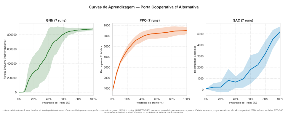
FIGURA 6.11. Curvas de aprendizagem no cenário Porta Cooperativa com Alternativa ( deceptive ).
