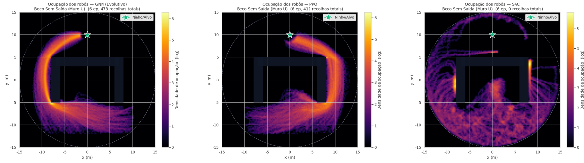
FIGURA 6.4. Densidade de ocupação dos robôs no Muro U (GNN, PPO e SAC, da esquerda para a direita; 6 episódios por painel, escala logarítmica). O GNN contorna a barra do U pela esquerda e o PPO pela direita — em ambos, um fluxo contínuo até ao ninho, com 473 e 412 recolhas. O SAC não resolve o cenário: a ocupação concentra-se colada às faces interiores das paredes verticais, o padrão de agentes presos, e o episódio termina com 0 recolhas . A escala de cor é normalizada por painel, pelo que as cores comparam a distribuição dentro de cada algoritmo, não a magnitude entre eles.
