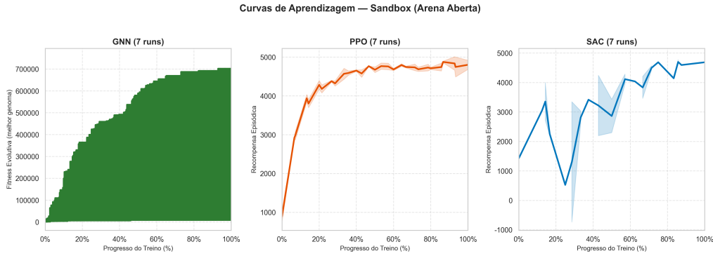
FIGURA 6.5. Curvas de aprendizagem dos três algoritmos no cenário Sandbox. O eixo das abcissas está normalizado (0–100% do orçamento de treino); linha = média de 7 runs , banda = \pm 1 desvio padrão.
