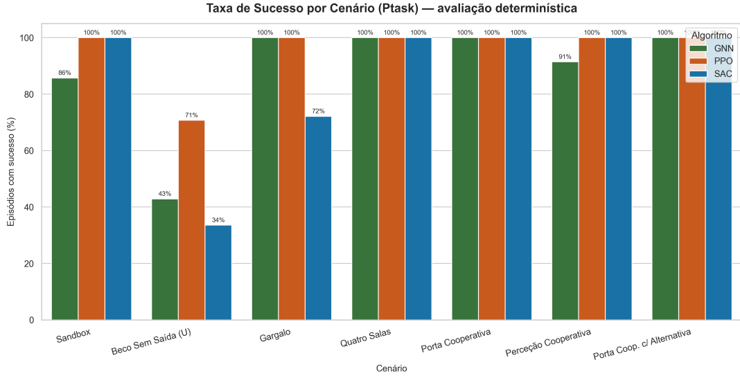
FIGURA 6.1. Taxa de sucesso ( P_{task} ) por cenário, em avaliação determinística ( 7 \text{ runs} \times 20 episódios emparelhados por algoritmo).
