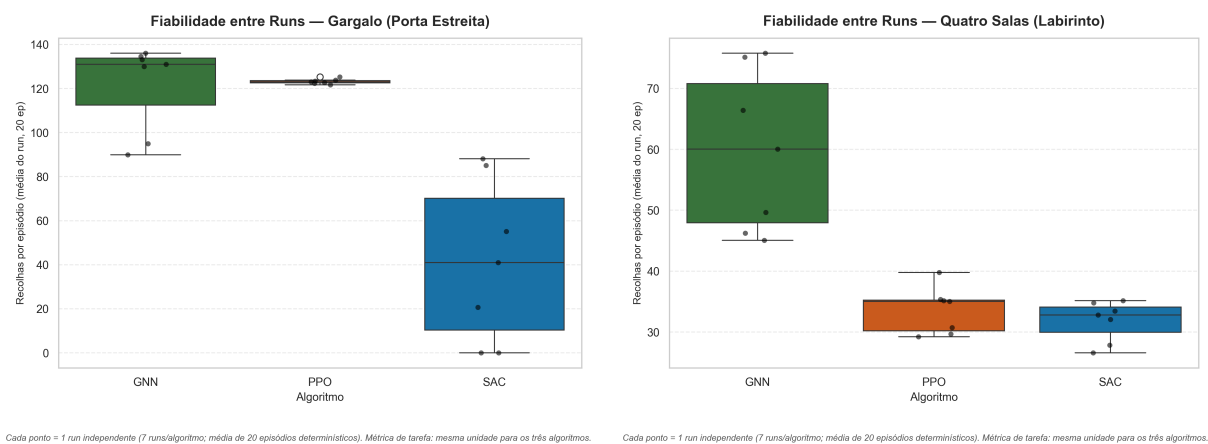
FIGURA 6.13. Recolhas/ep por run : Gargalo (esq.) e Quatro Salas (dir.).
