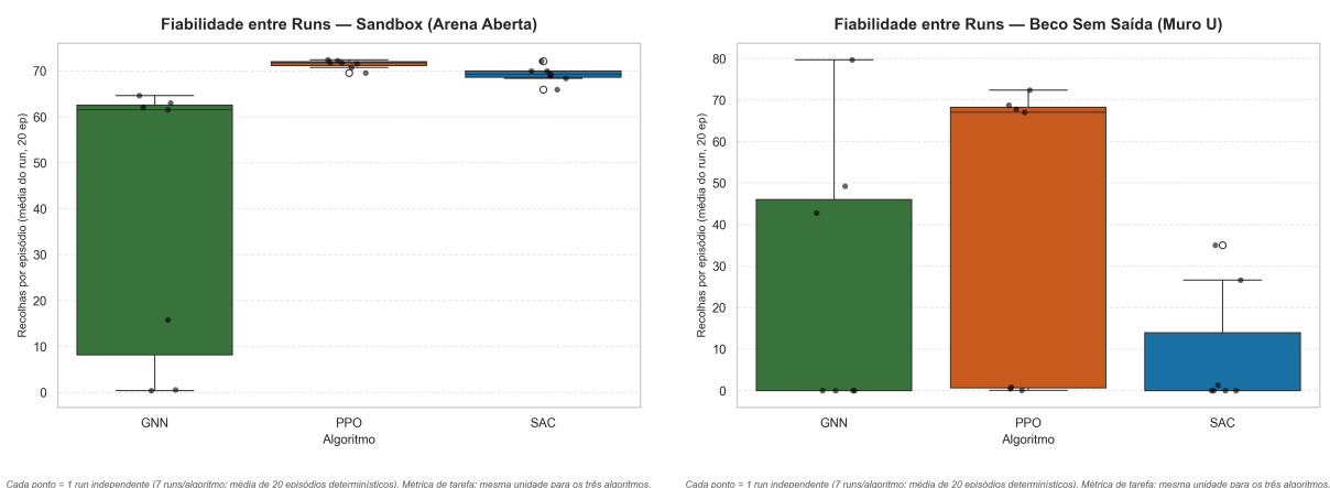
FIGURA 6.12. Recolhas/ep por run (7 runs , 20 ep cada): Sandbox (esq.) e Muro U (dir.).
