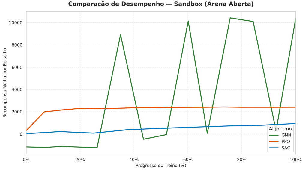
FIGURA 6.5. Curvas de aprendizagem dos três algoritmos no cenário Sandbox. O eixo das abcissas está normalizado (0–100% do treino). Cada curva corresponde a uma única execução de treino (ver Secção 6.6).
