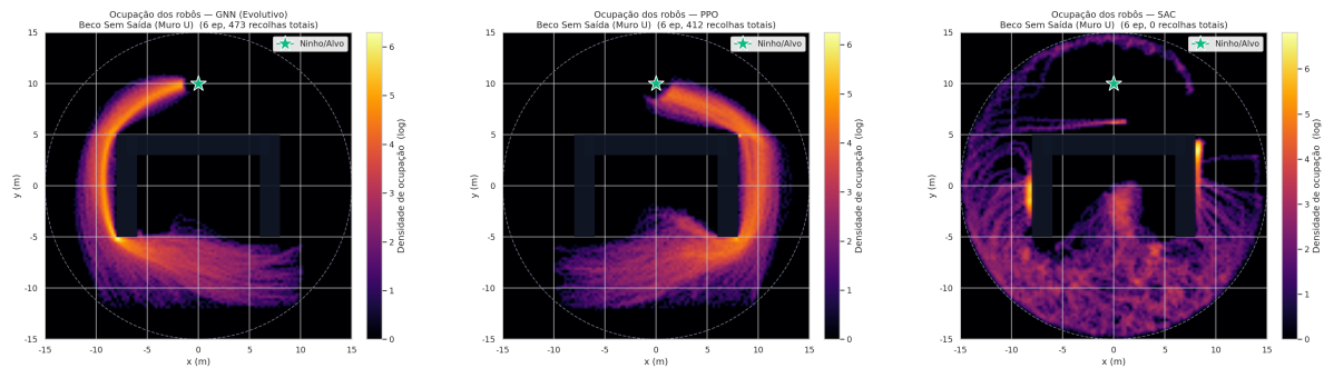
FIGURA 6.4. Densidade de ocupação dos robôs no Muro em U (GNN, PPO e SAC, da esquerda para a direita; 6 episódios por painel, escala logarítmica). O GNN contorna a barra do U pela esquerda e o PPO pela direita — em ambos, um fluxo contínuo até ao ninho, com 473 e 412 recolhas. O SAC não resolve o cenário: a ocupação concentra-se colada às faces interiores das paredes verticais, o padrão de agentes presos, e o episódio termina com 0 recolhas . A escala de cor é normalizada por painel, pelo que as cores comparam a distribuição dentro de cada algoritmo, não a magnitude entre eles.
