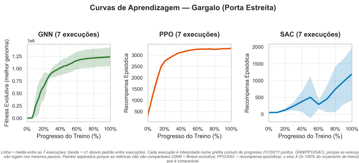
FIGURA 6.7. Curvas de aprendizagem no cenário Gargalo.
