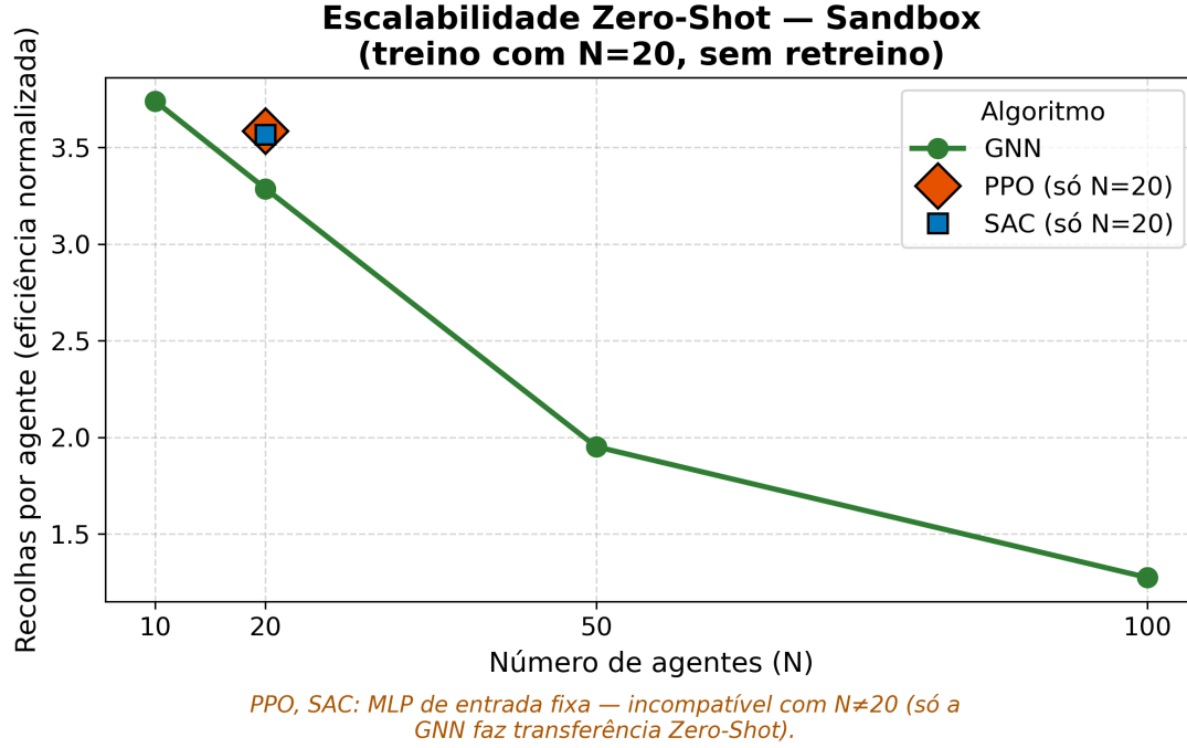
FIGURA 6.24. Eficiência por agente (recolhas por episódio a dividir pelo número de agentes) com o aumento do enxame, sem retreino, no cenário Sandbox. Só a linha do controlador de grafo atravessa toda a gama: o PPO e o SAC têm um único ponto, em N = 20 (o losango e o quadrado de contorno preto, sobrepostos porque distam 0,02 recolhas por agente), porque a política MLP de entrada fixa não admite outras dimensões de enxame.
