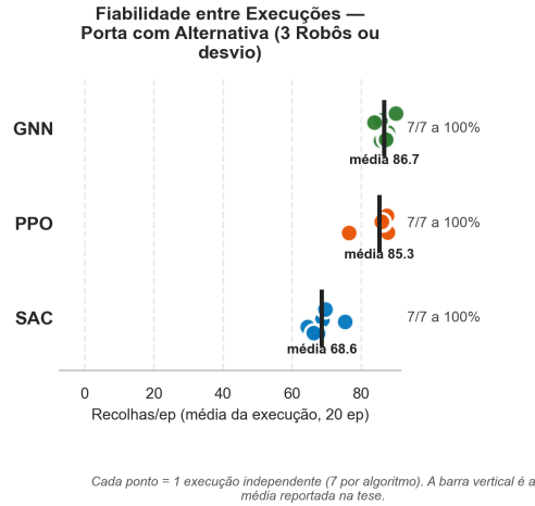
FIGURA 6.15. Recolhas/ep por execução: Porta Cooperativa com Alternativa ( deceptive ).
