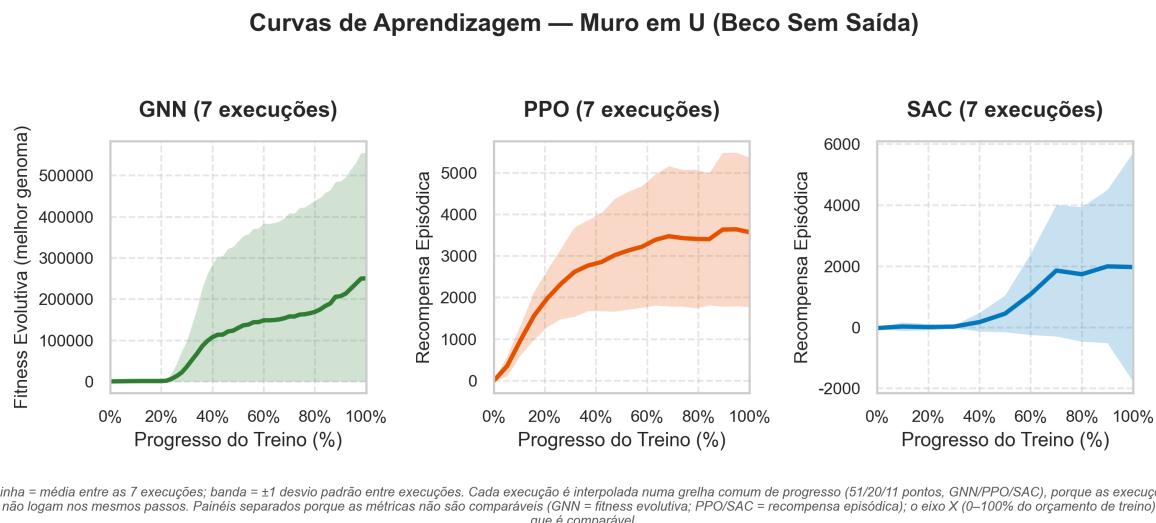
FIGURA 6.6. Curvas de aprendizagem no cenário Beco Sem Saída (Muro em U).
