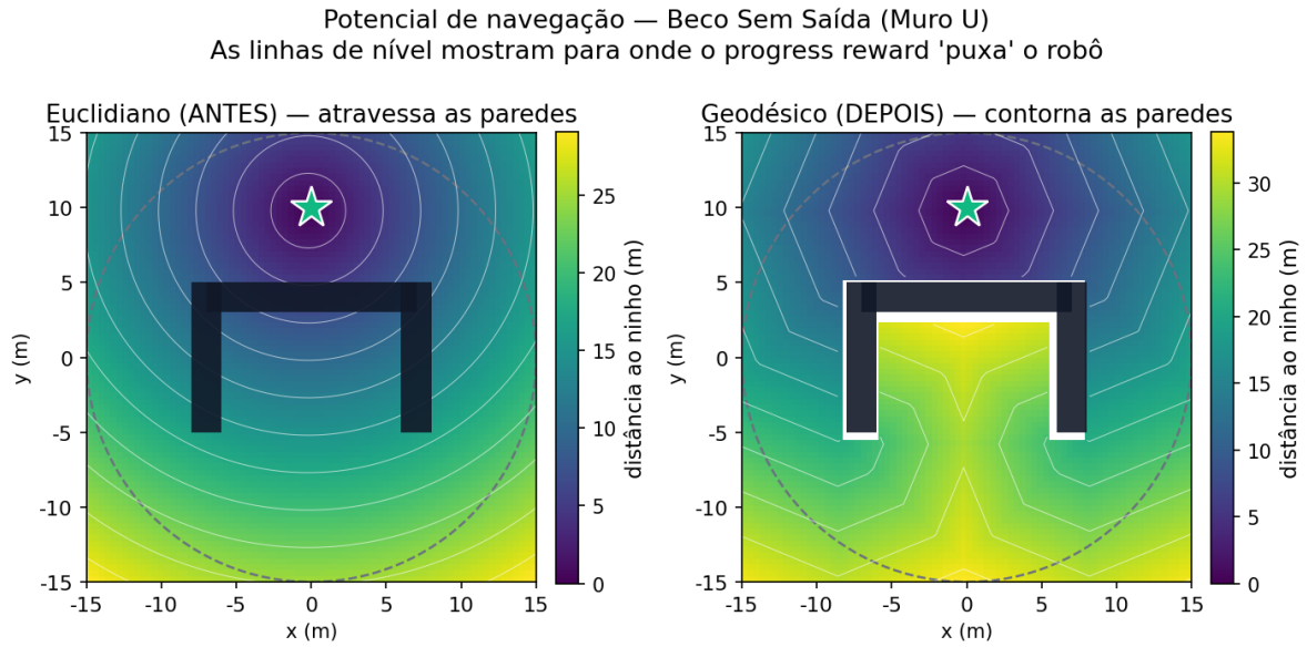
FIGURA 6.3. Potencial de navegação no Muro em U: euclidiano (esquerda) vs. geodésico (direita). As curvas de nível indicam a direção para a qual o termo de progresso atrai o agente; só o geodésico contorna a barra do U.
