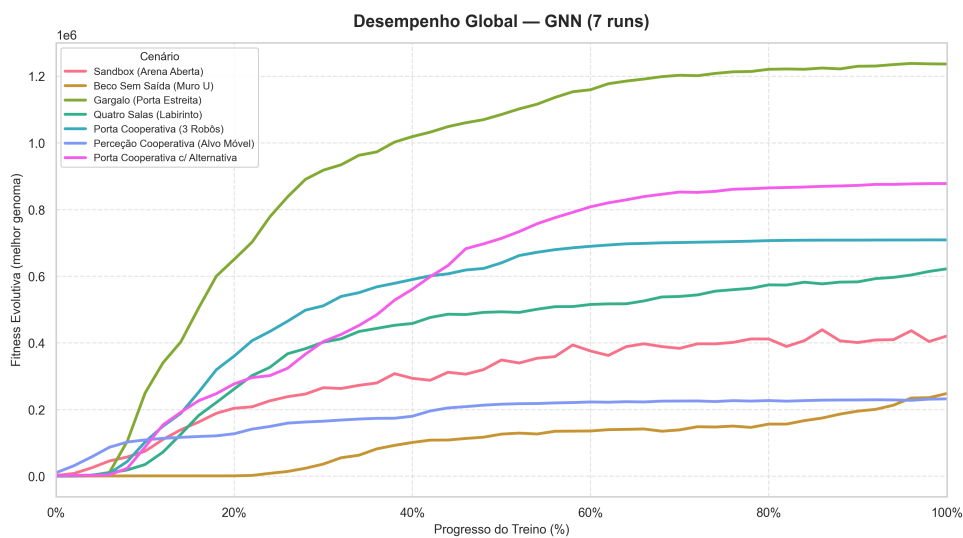
FIGURA 6.16. Desempenho do GNN (evolutivo) nos sete cenários (linha = média entre os 7 runs por progresso de treino).
