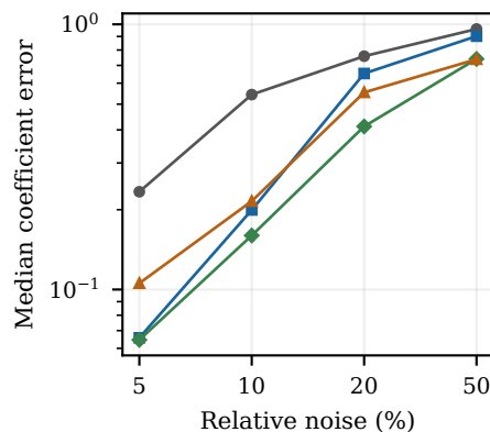
Advection-diffusion
