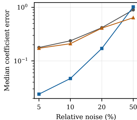
Advection-diffusion
