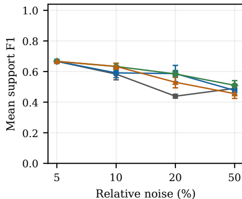
Advection-diffusion
