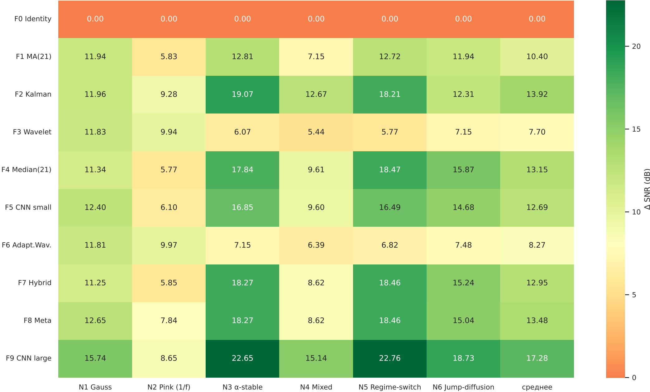
Прирост SNR (дБ): все 10 фильтров × 6 шумов; столбец «среднее» итожит универсальность
