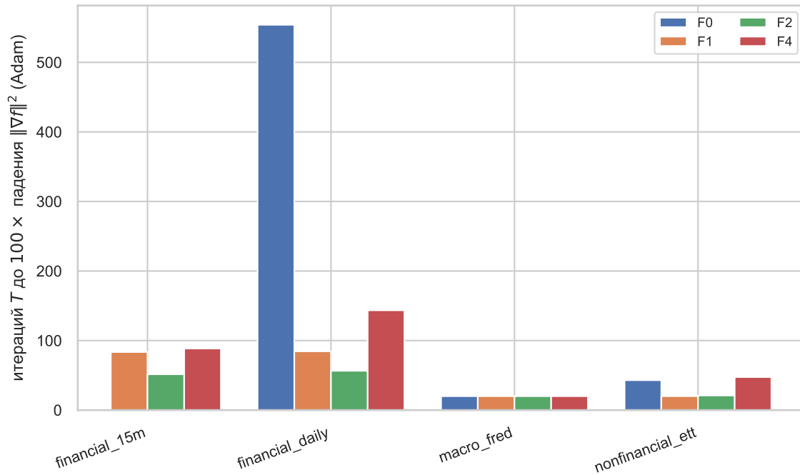
(а) Время сходимости по доменам (ниже — быстрее; не сошедшиеся опущены)
