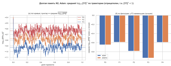
Рис. 4: Та же конфигурация (N2, Adam). Слева — кривые \log_{10} \|\nabla f\|^2 , пунктир — их среднее по траектории ( \log_{10} \|\nabla f\|^2 ). Справа — это среднее по фильтрам: оно отрицательно, потому что \|\nabla f\|^2 < 1 даёт отрицательный логарифм; у F3 оно наименьшее (наилучшее).
