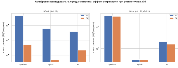
Рис. 5: Синтетика, откалиброванная под реальные \hat{\alpha} и \hat{d} . При тяжёлохвостовом N3cal разрыв F0/F4 сохраняется (91–120×). При смешанном N4cal разрыва нет.
