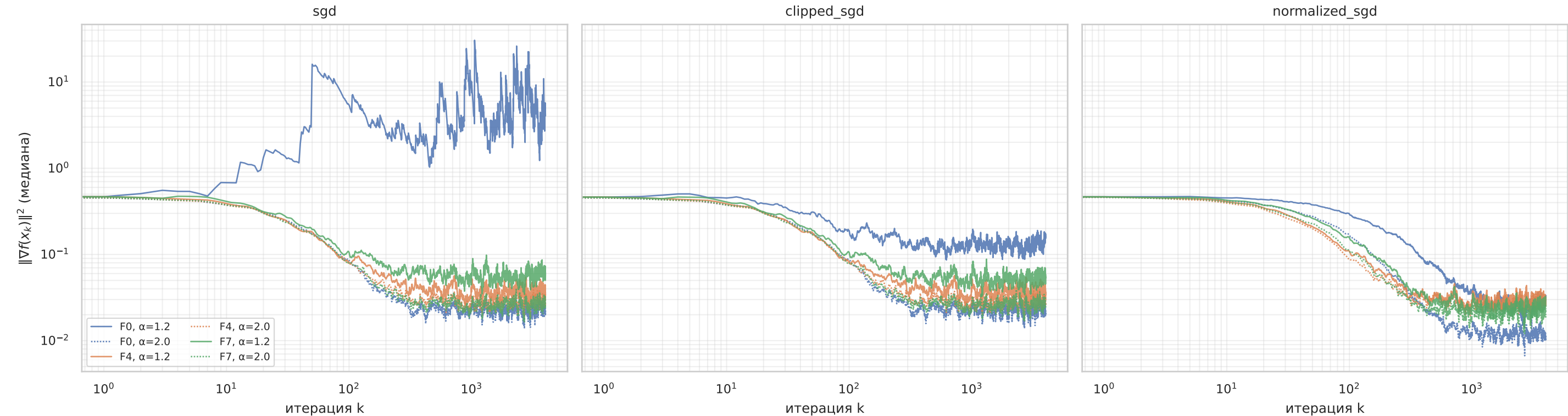
Сходимость на квадратичной задаче при разных \alpha (heavy-tail) и фильтрах
