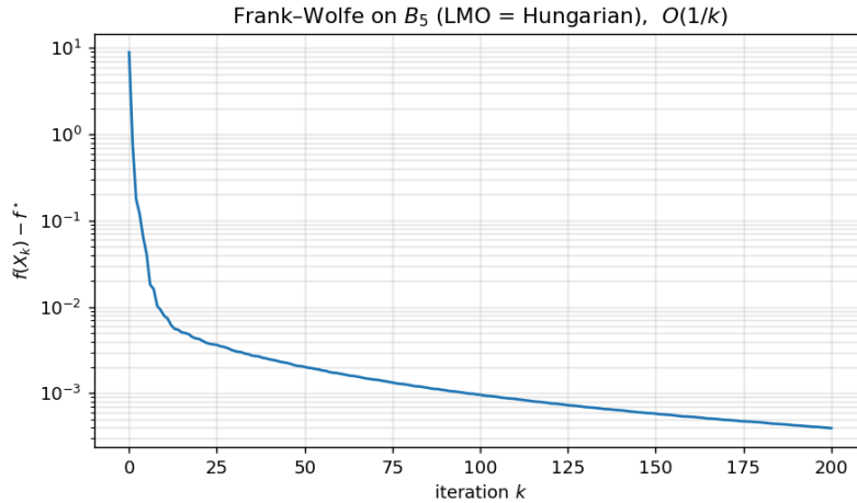
Рис. 6. Франк–Вульф на B_5 , LMO = венгерский алгоритм, скорость O(1/k) .
