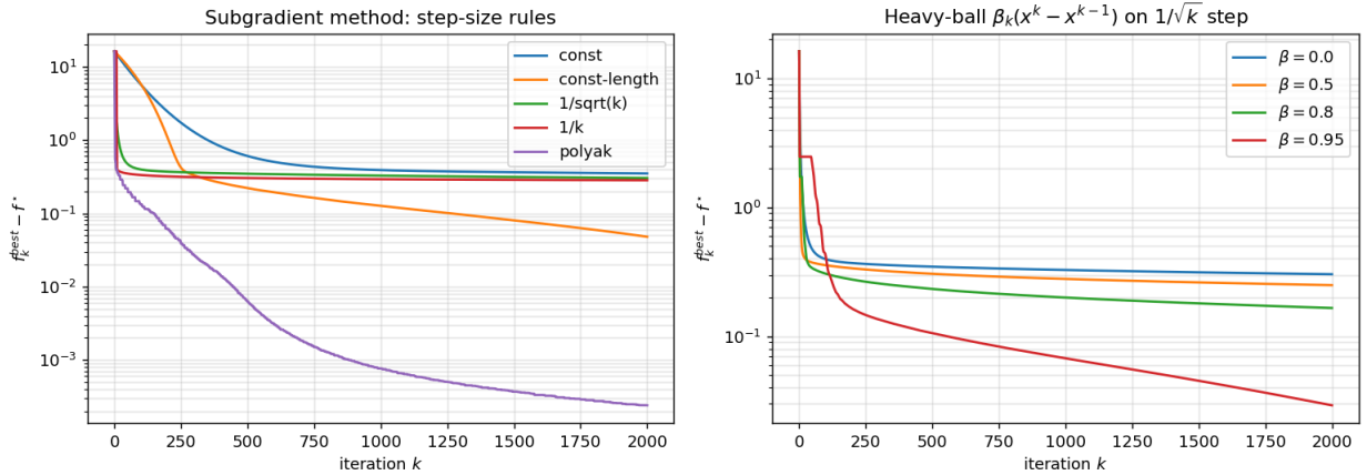
Рис. 9. LASSO: правила выбора шага (слева) и тяжёлый шар (справа).
