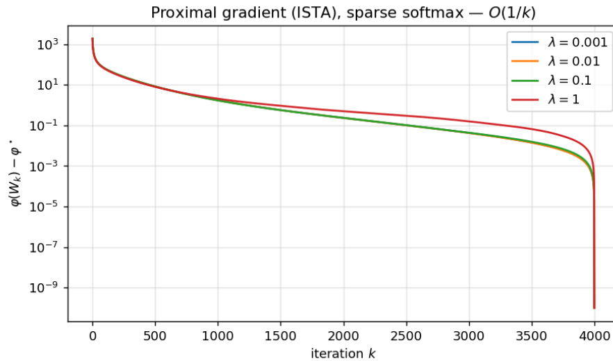
Рис. 11. Проксимальный градиент (ISTA), \phi(W_k) - \phi^* , скорость O(1/k) .
