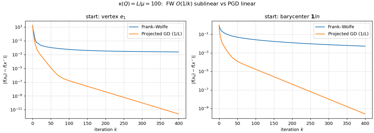
Рис. 7. Квадратичная задача на \Delta_{20} : FW O(1/k) против линейного PGD.
