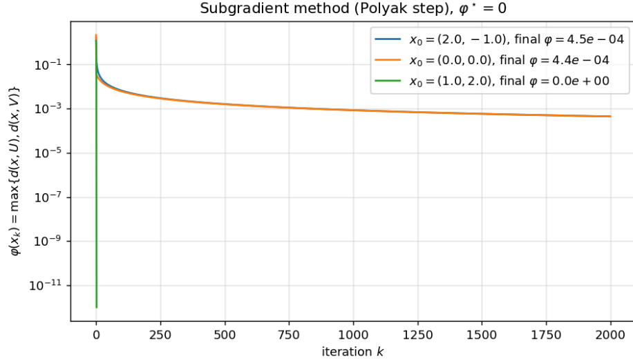
Рис. 8. Субградиентный метод (шаг Поляка), \phi^* = 0 ; разные старты.
