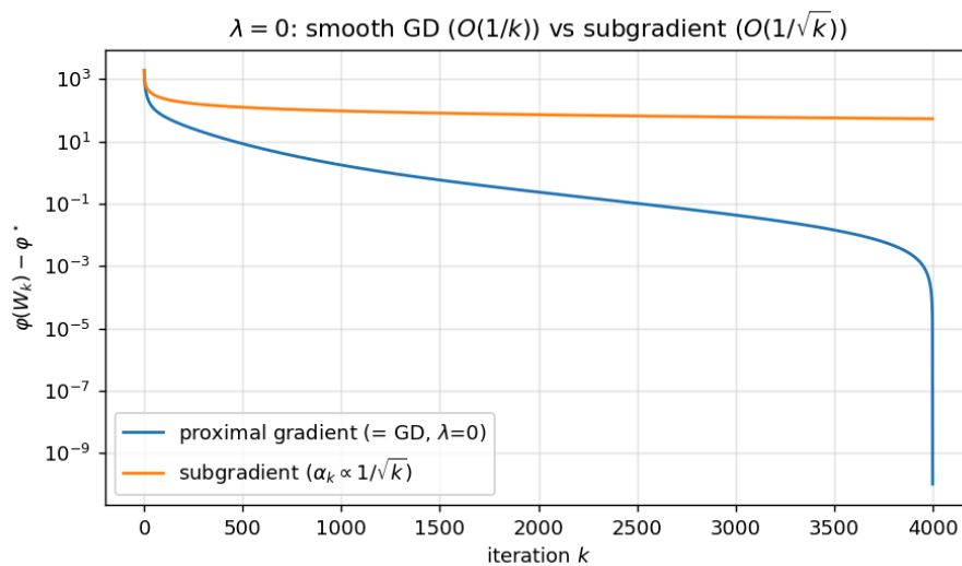
Рис. 10. \lambda = 0 : проксимальный (= GD, O(1/k) ) против субградиента ( O(1/\sqrt{k}) ).
