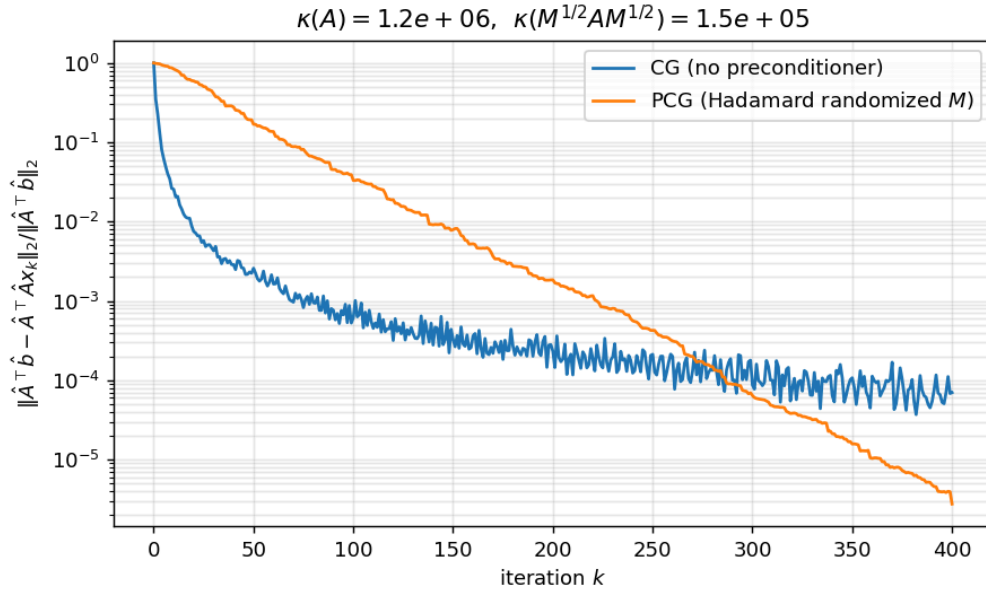
Рис. 1. Относительная невязка \|\hat{A}^\top \hat{b} - \hat{A}^\top \hat{A} x_k\|_2 / \|\hat{A}^\top \hat{b}\|_2 .
