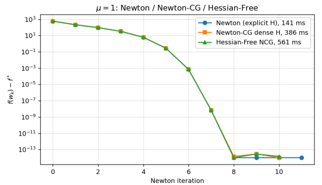
Рис. 5. (f,g) Ньютон / Ньютон–CG / HFN.
