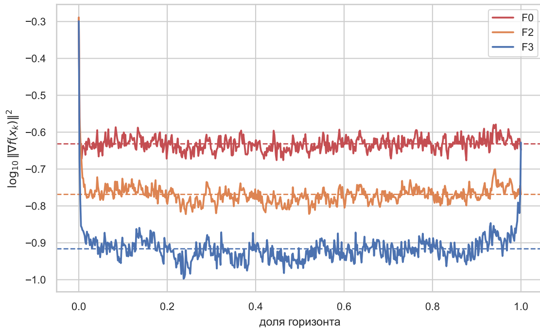
(а) лог-кривые; пунктир — среднее \log_{10} \|\nabla f\|^2
