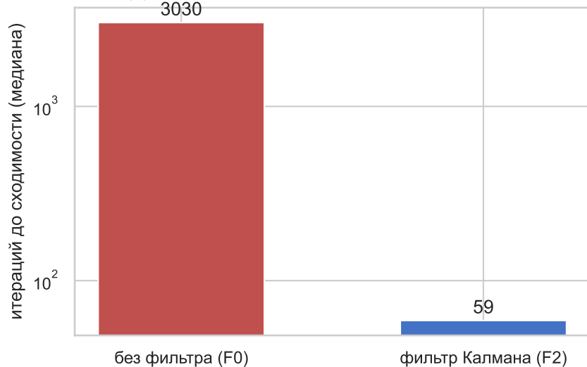
(а) скорость: фильтр сходится в ~50 раз быстрее
