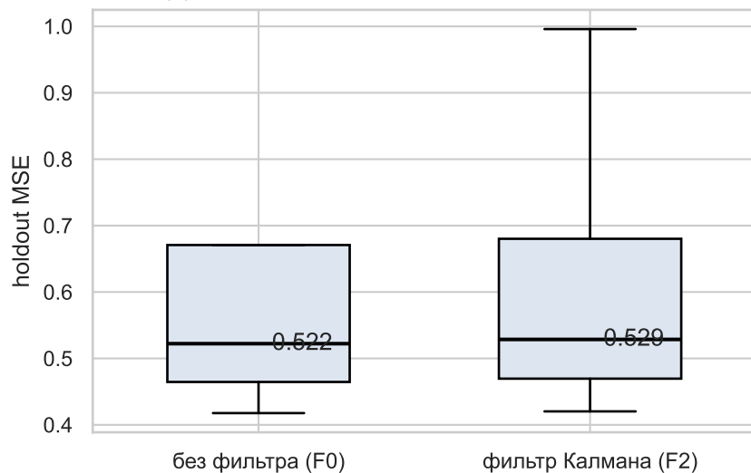
(б) точность: holdout-MSE практически одинаков
