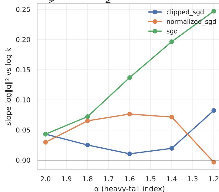
(d) F0 convergence slope vs \alpha — SGD diverges at \alpha=1.2
