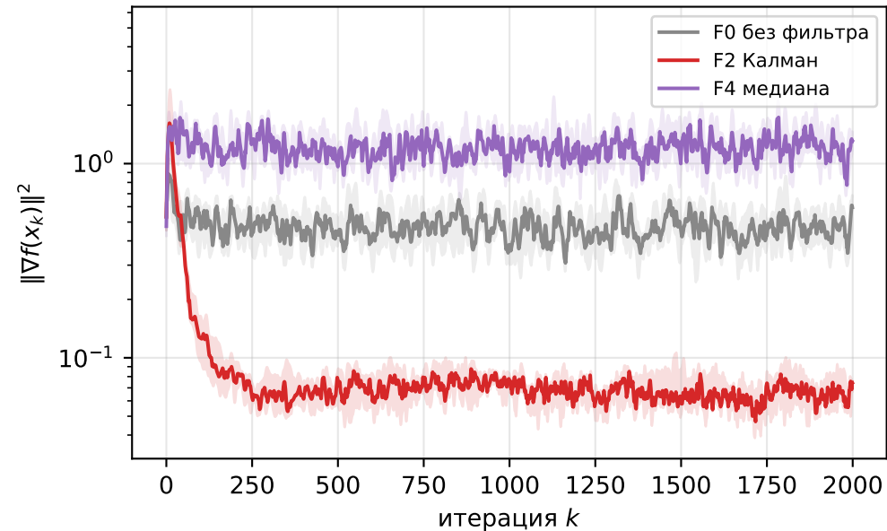
Квадратичная задача, Adam, N1 гаусс
