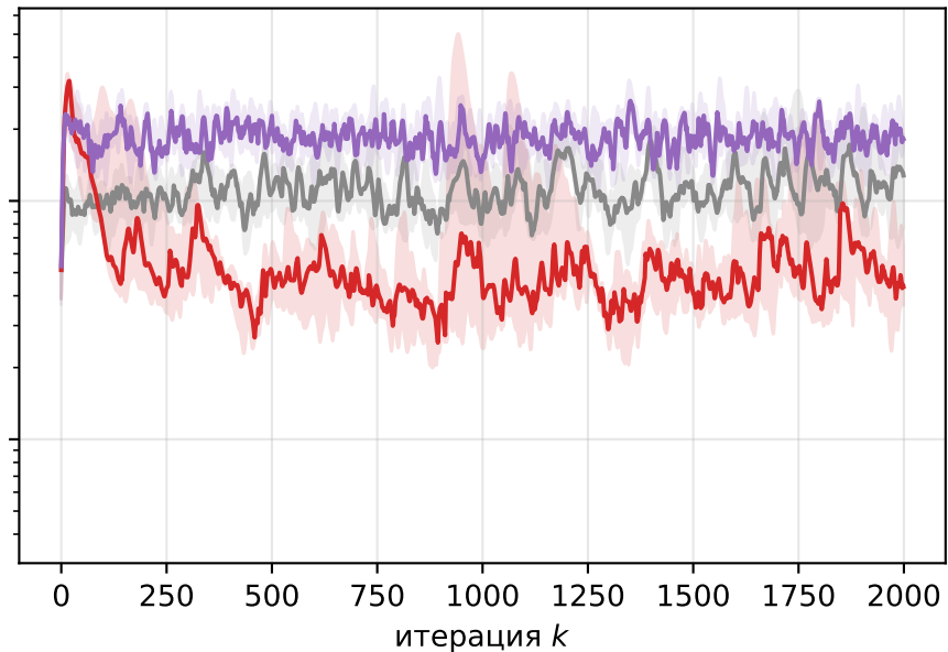
Квадратичная задача, Adam, N3 тяжёлый
