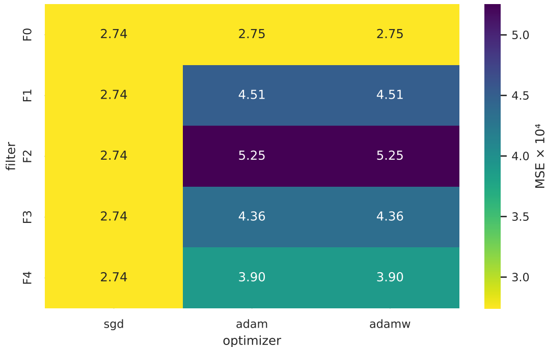
Реальные данные: holdout MSE по парам (фильтр, оптимизатор)
